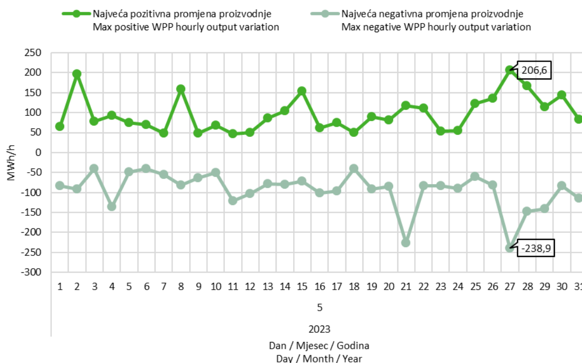
Slika 9 Maksimalna pozitivna i maksimalna negativna promjena satne proizvodnje VE u svibnju 2023. godine
