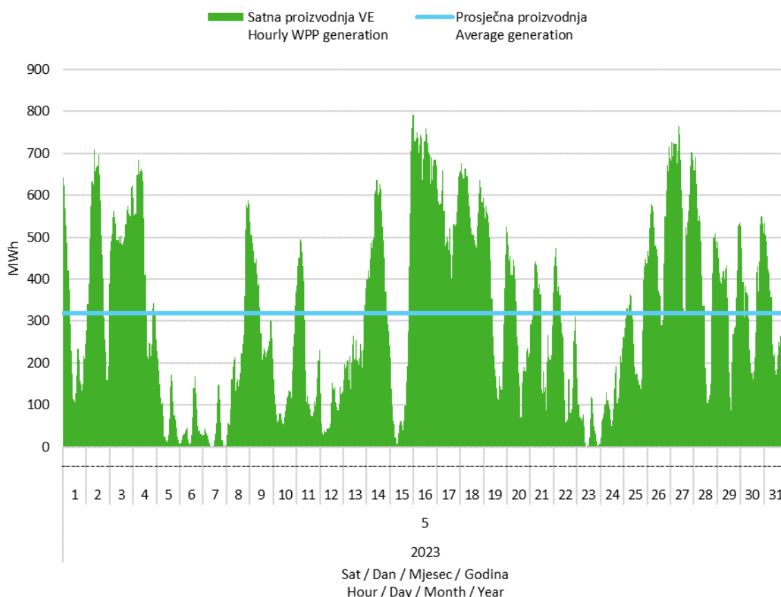
Slika 2 Satna proizvodnja svih vjetroelektrana u svibnju 2023. godine
