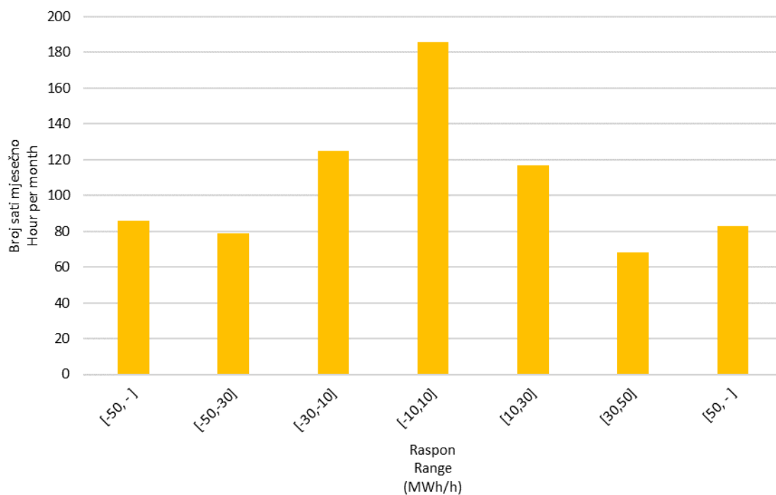
Slika 10 Statistička raspodjela satnih promjena proizvodnje VE u svibnju 2023. godine
