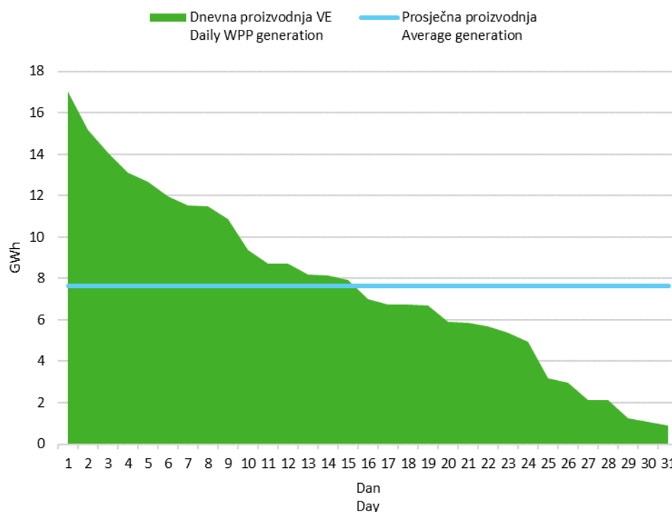
Slika 6 Krivulja trajanja dnevne proizvodnje vjetroelektrana u svibnju 2023. godine
