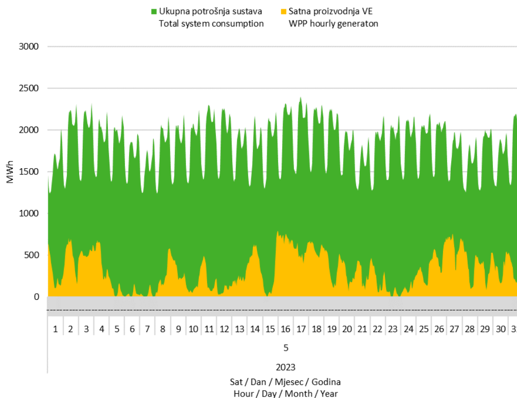
Slika 7 Usporedba satnog dijagrama opterećenja sustava i proizvodnje vjetroelektrana u svibnju 2023. godine
