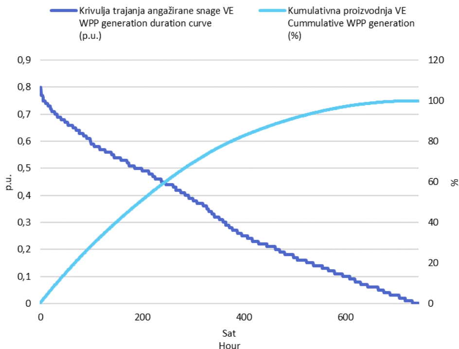
Slika 3 Krivulja trajanja angažirane snage svih VE i kumulativna proizvodnja VE u svibnju 2023. godine u jediničnim vrijednostima
