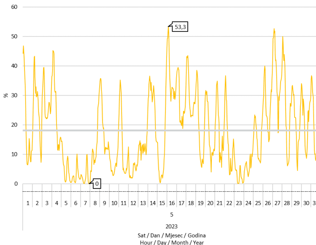
Slika 8 Udio proizvodnje vjetroelektrana u pokrivanju satnog opterećenja elektroenergetskog sustava u svibnju 2023. godine
