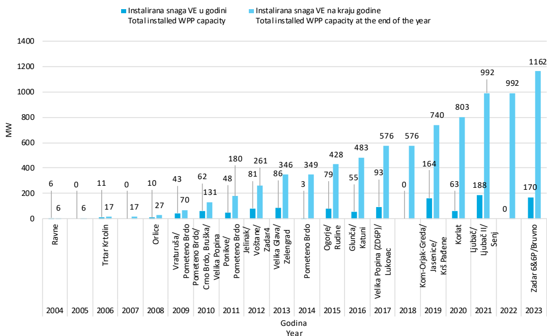
Slika 2 Vremenska dinamika izgradnje VE u Hrvatskoj
