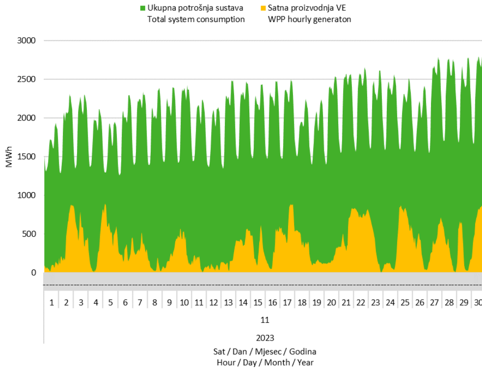
Slika 7 Usporedba satnog dijagrama opterećenja sustava i proizvodnje vjetroelektrana u studenom 2023. godine
