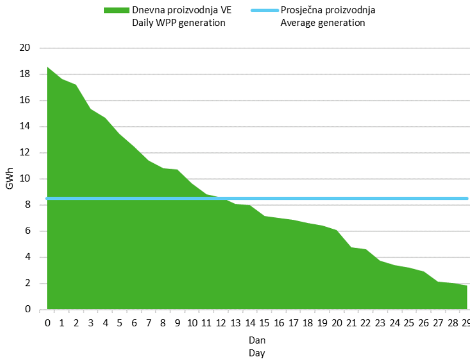
Slika 6 Krivulja trajanja dnevne proizvodnje vjetroelektrana u studenom 2023. godine
