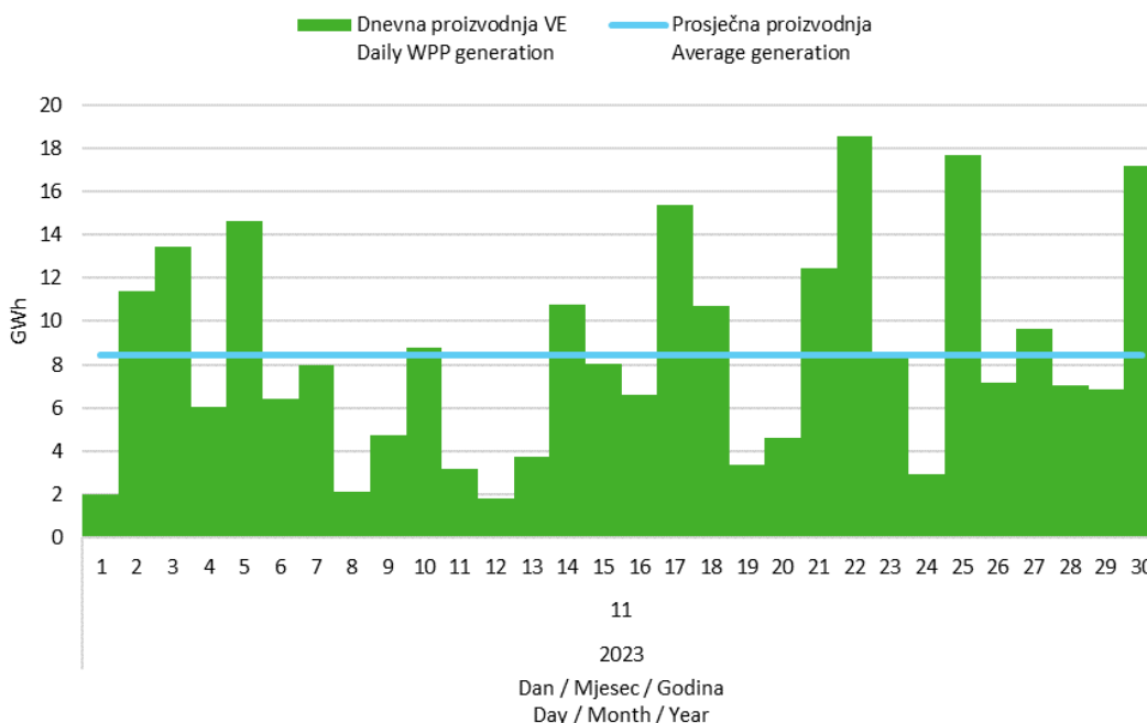
Slika 5 Dnevna proizvodnja svih vjetroelektrana u studenom 2023. godine Figure 5 Daily generation of all wind power plants in November 2023
