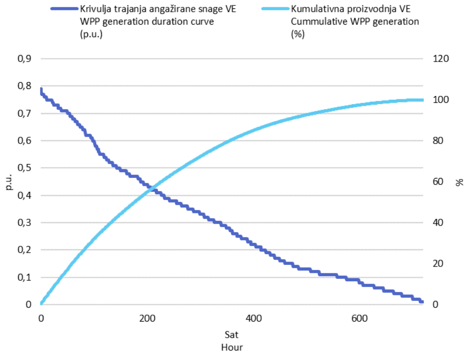
Slika 3 Krivulja trajanja angažirane snage svih VE i kumulativna proizvodnja VE u studenom 2023. godine u jediničnim vrijednostima
