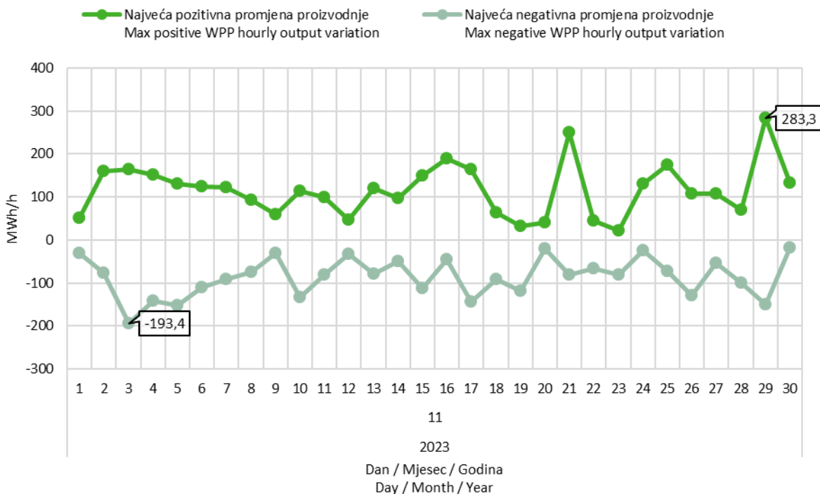
Slika 9 Maksimalna pozitivna i maksimalna negativna promjena satne proizvodnje VE u studenom 2023. godine
