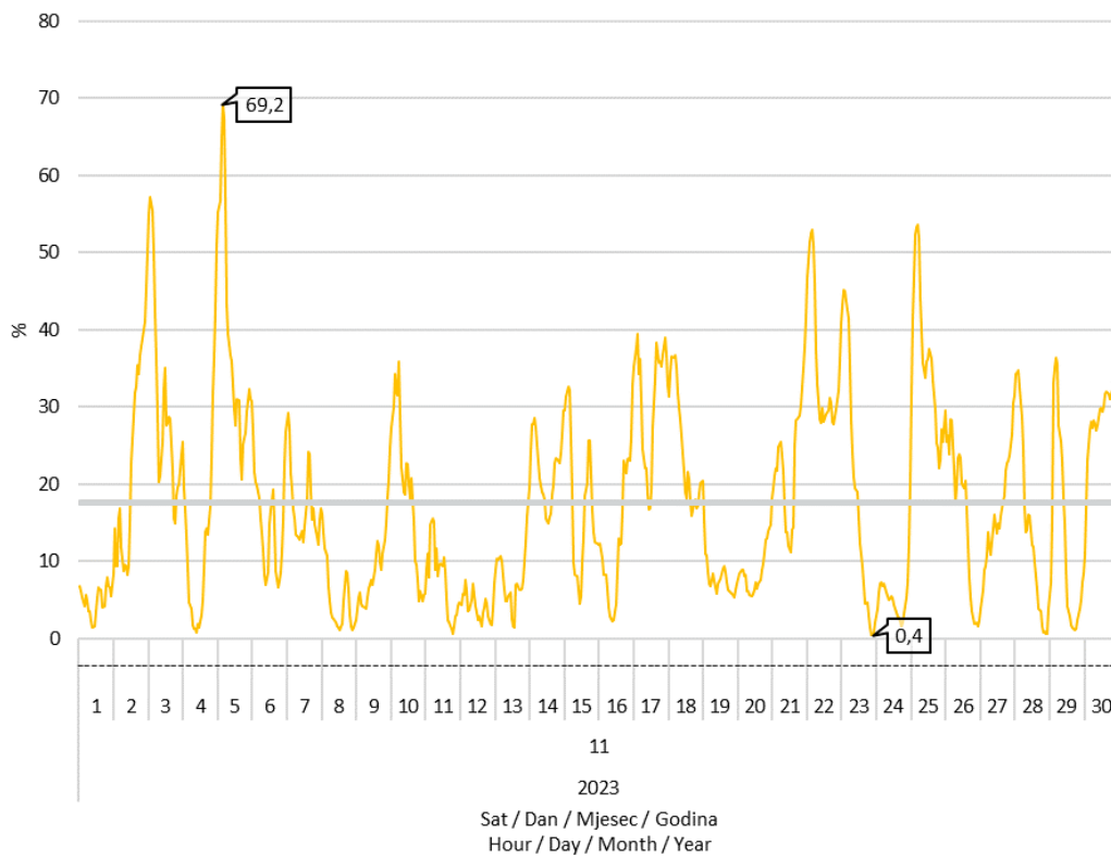
Slika 8 Udio proizvodnje vjetroelektrana u pokrivanju satnog opterećenja elektroenergetskog sustava u studenom 2023. godine
