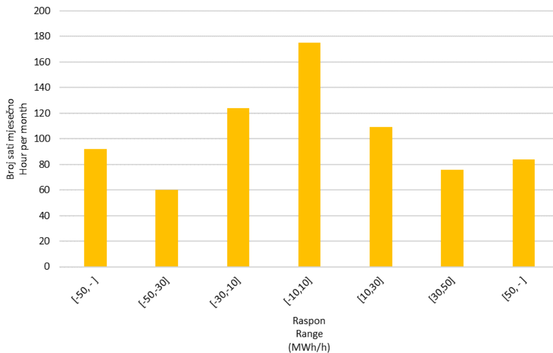
Slika 10 Statistička raspodjela satnih promjena proizvodnje VE u studenom 2023. godine
