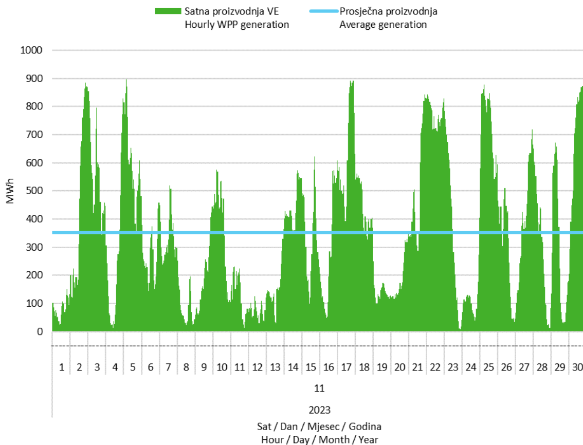
Slika 2 Satna proizvodnja svih vjetroelektrana u studenom 2023. godine
