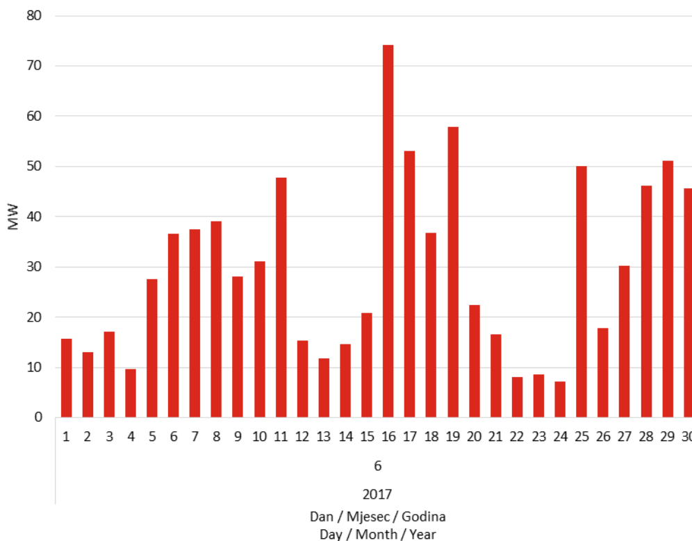
Slika 15 Korijen srednje kvadratne pogreške prognoze satne proizvodnje svih VE u lipnju 2017. godine
