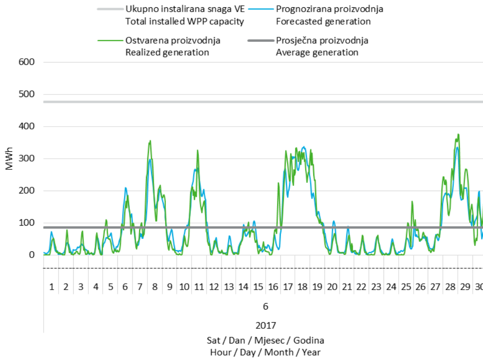
Slika 11 Prognozirana i ostvarena satna proizvodnja vjetroelektrana u lipnju 2017. godine
