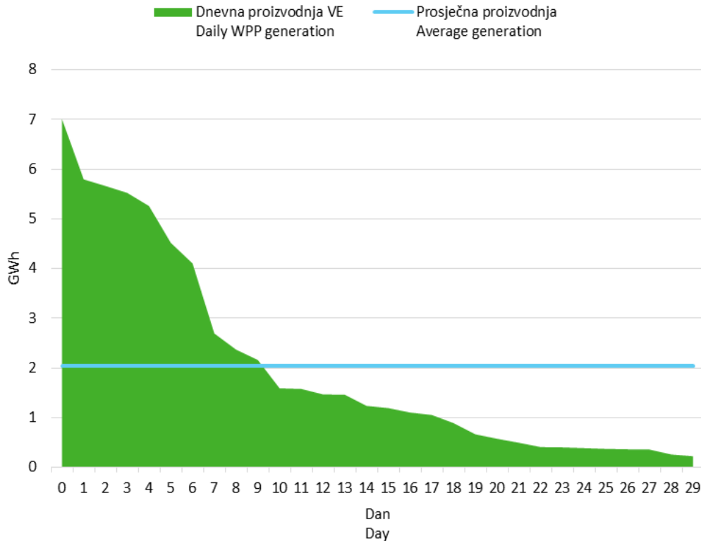
Slika 6 Krivulja trajanja dnevne proizvodnje vjetroelektrana u lipnju 2017. godine
