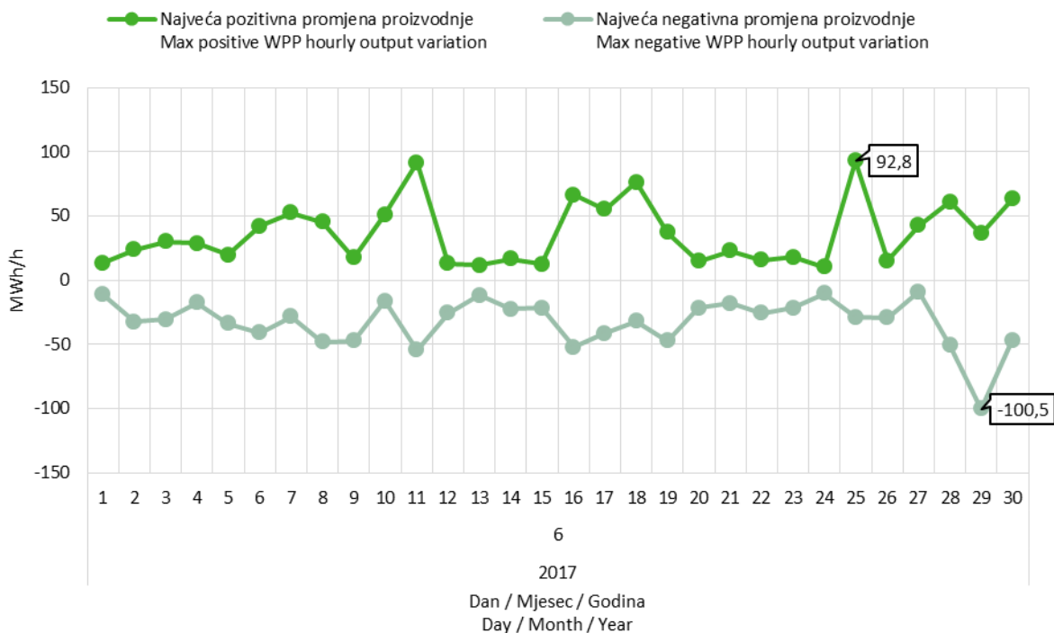
Slika 9 Maksimalna pozitivna i maksimalna negativna promjena satne proizvodnje VE u lipnju 2017. godine
