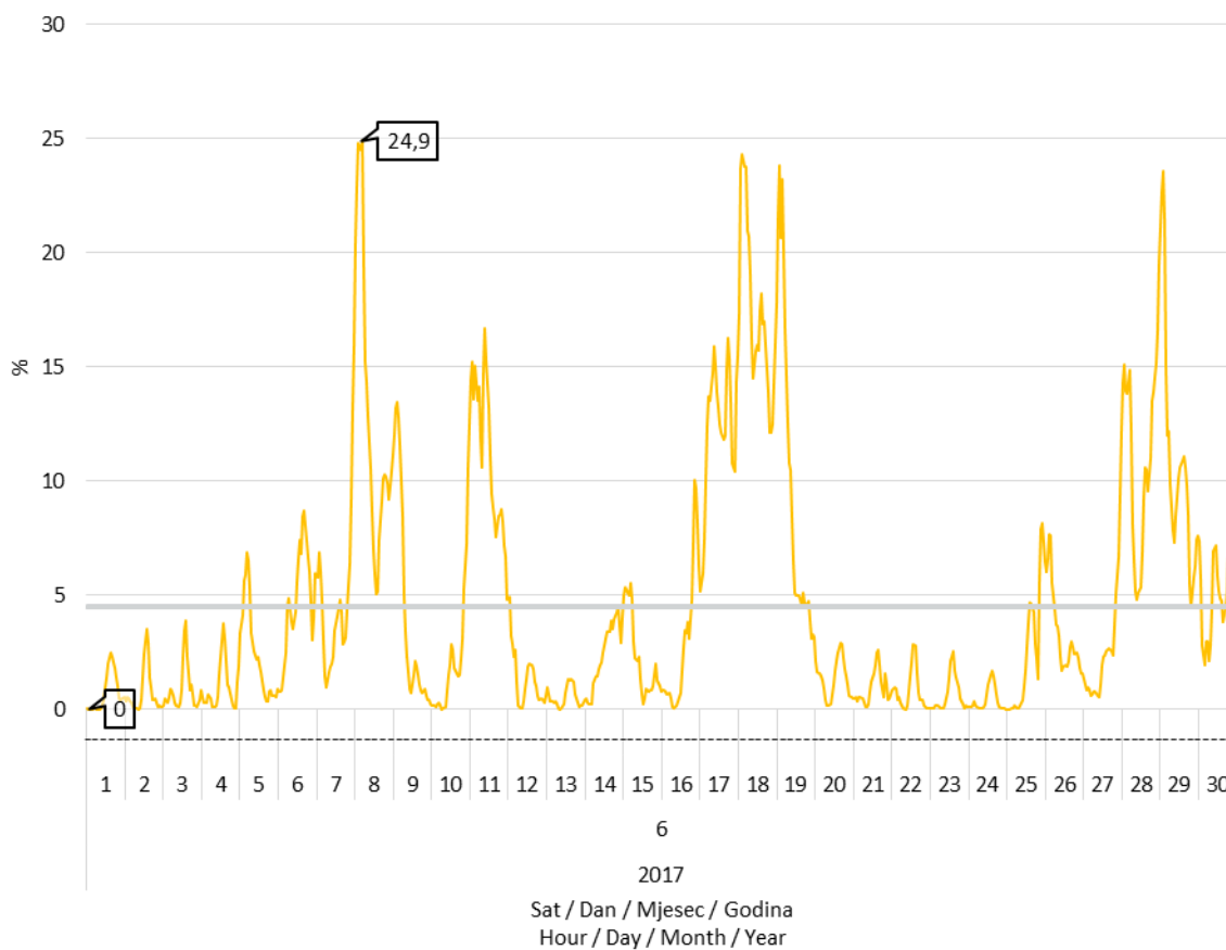
Slika 8 Udio proizvodnje vjetroelektrana u pokrivanju satnog opterećenja elektroenergetskog sustava u lipnju 2017. godine
