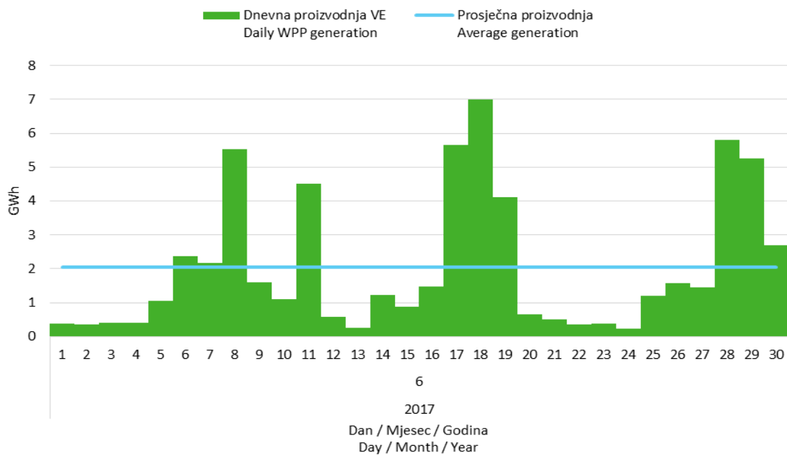
Slika 5 Dnevna proizvodnja svih vjetroelektrana u lipnju 2017. godine
