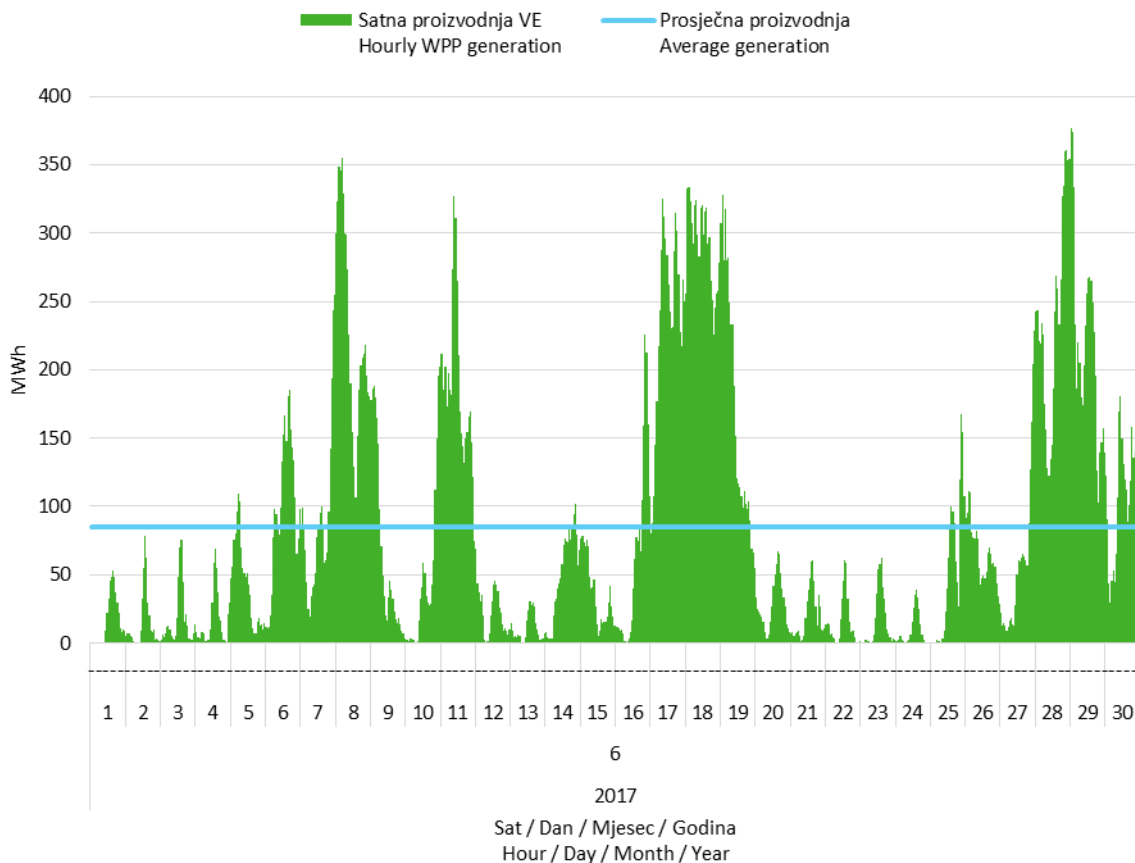
Slika 2 Satna proizvodnja svih vjetroelektrana u lipnju 2017. godine
