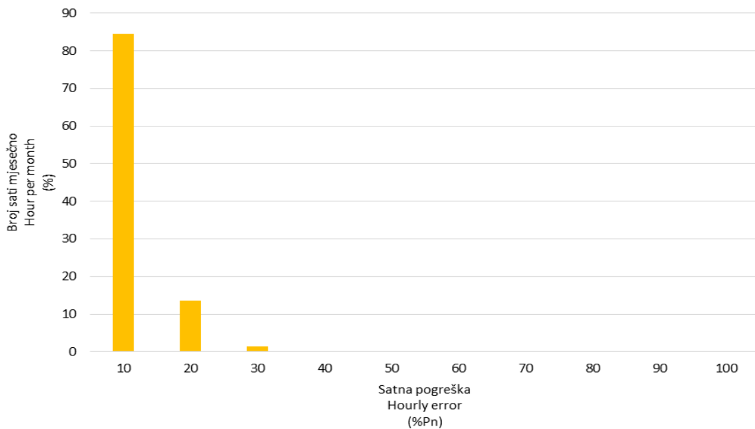
Slika 17 Frekvencija pojavljivanja pogreške prognoze satne proizvodnje svih VE u lipnju 2017. godine
