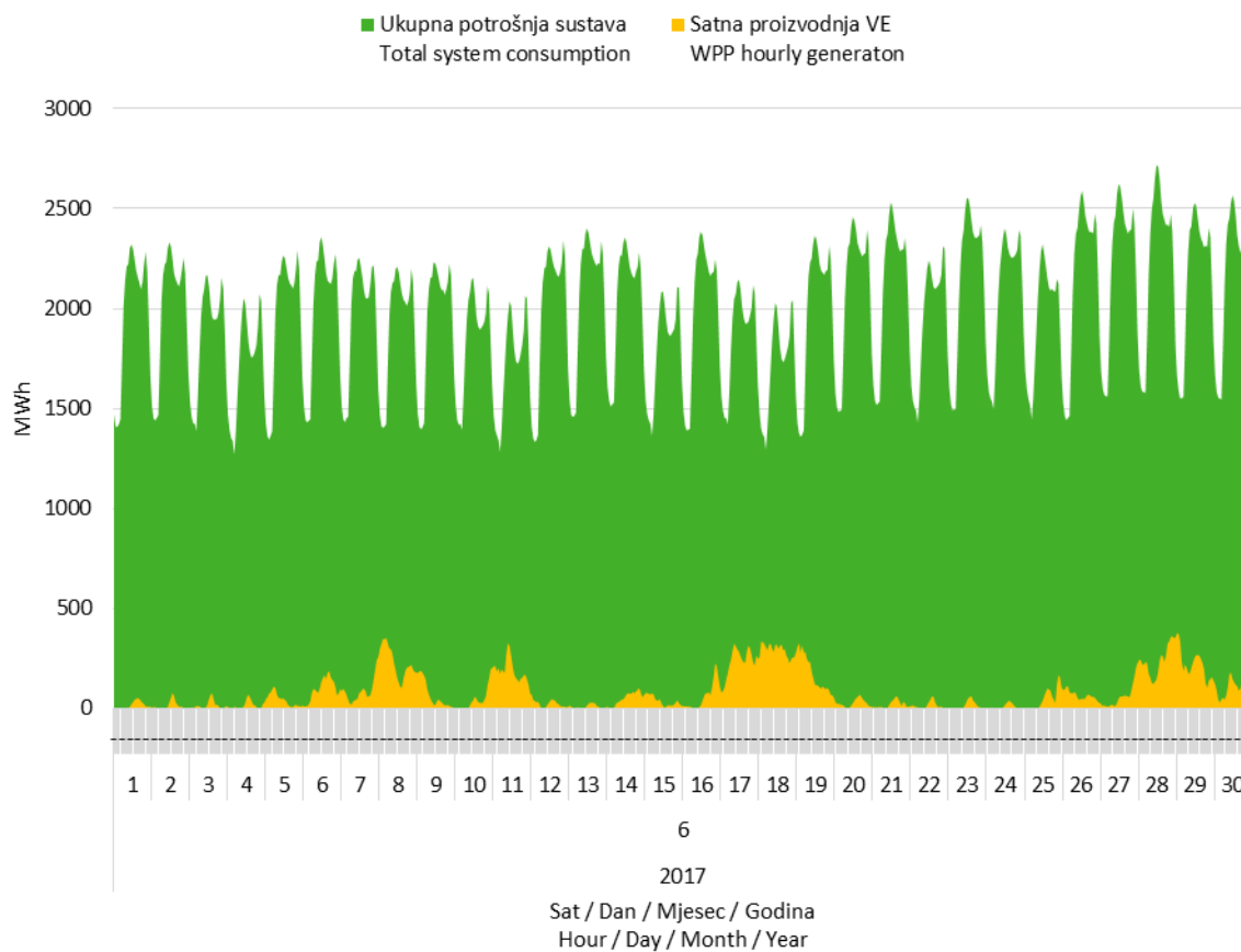
Slika 7 Usporedba satnog dijagrama opterećenja sustava i proizvodnje vjetroelektrana u lipnju 2017. godine
