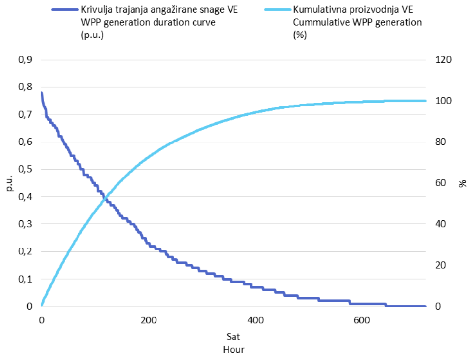
Slika 3 Krivulja trajanja angažirane snage svih VE i kumulativna proizvodnja VE u lipnju 2017. godine u jediničnim vrijednostima
