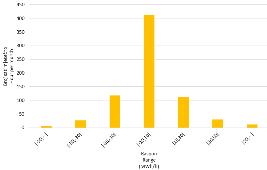
Slika 10 Statistička raspodjela satnih promjena proizvodnje VE u lipnju 2017. godine
