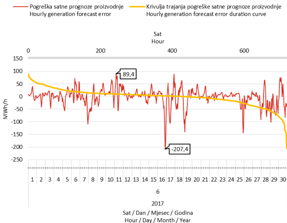
Slika 12 Razlika između prognozirane i ostvarene satne proizvodnje svih VE (pogreška prognoze) i pripadna krivulja trajanja u lipnju 2017. godine
