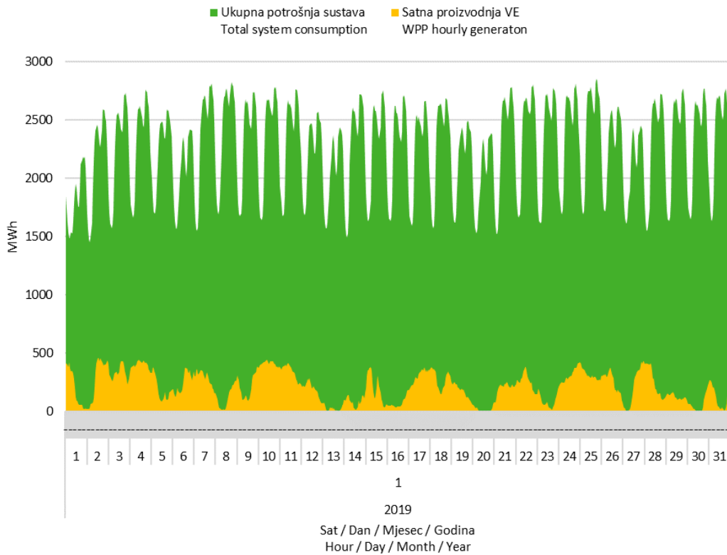
Slika 7 Usporedba satnog dijagrama opterećenja sustava i proizvodnje vjetroelektrana u siječnju 2019. godine
