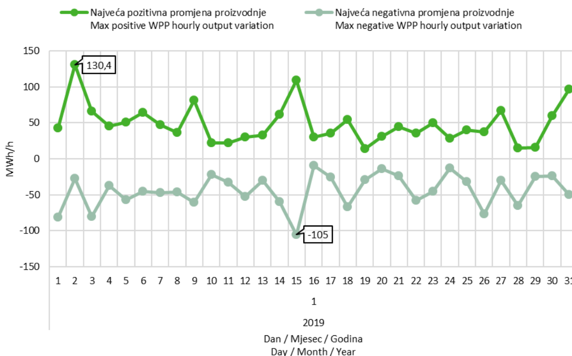
Slika 9 Maksimalna pozitivna i maksimalna negativna promjena satne proizvodnje VE u siječnju 2019. godine
