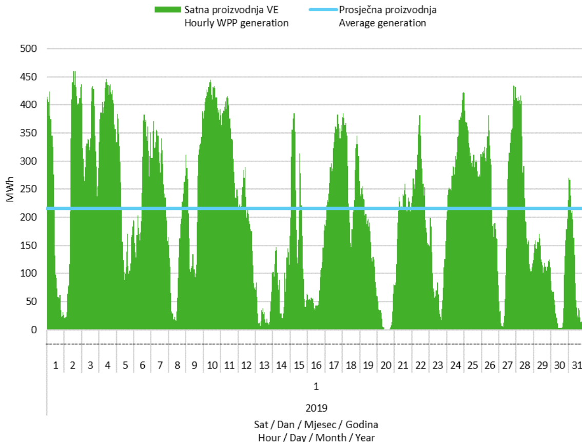
Slika 2 Satna proizvodnja svih vjetroelektrana u siječnju 2019. godine
