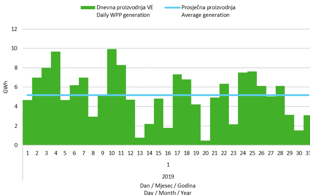
Slika 5 Dnevna proizvodnja svih vjetroelektrana u siječnju 2019. godine
