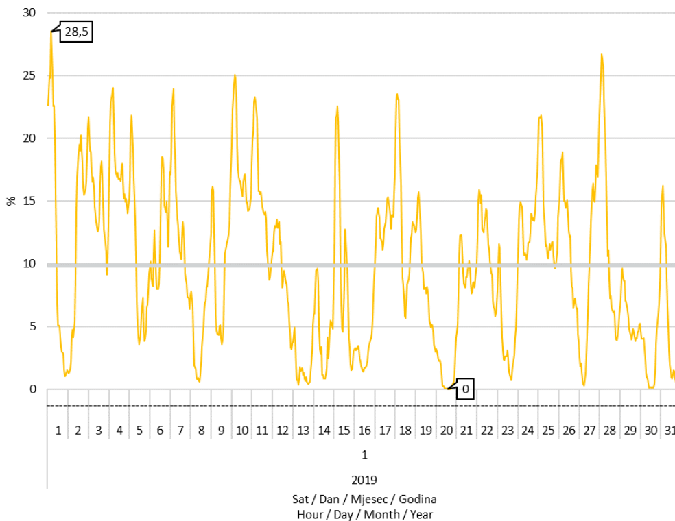
Slika 8 Udio proizvodnje vjetroelektrana u pokrivanju satnog opterećenja elektroenergetskog sustava u siječnju 2019. godine
