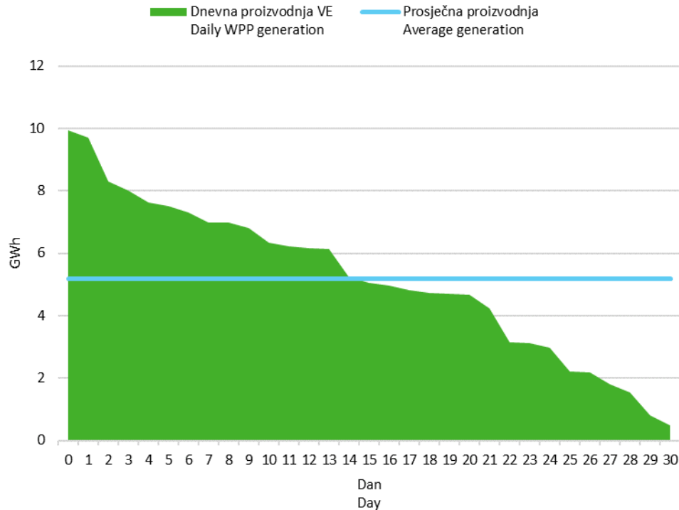
Slika 6 Krivulja trajanja dnevne proizvodnje vjetroelektrana u siječnju 2019. godine
