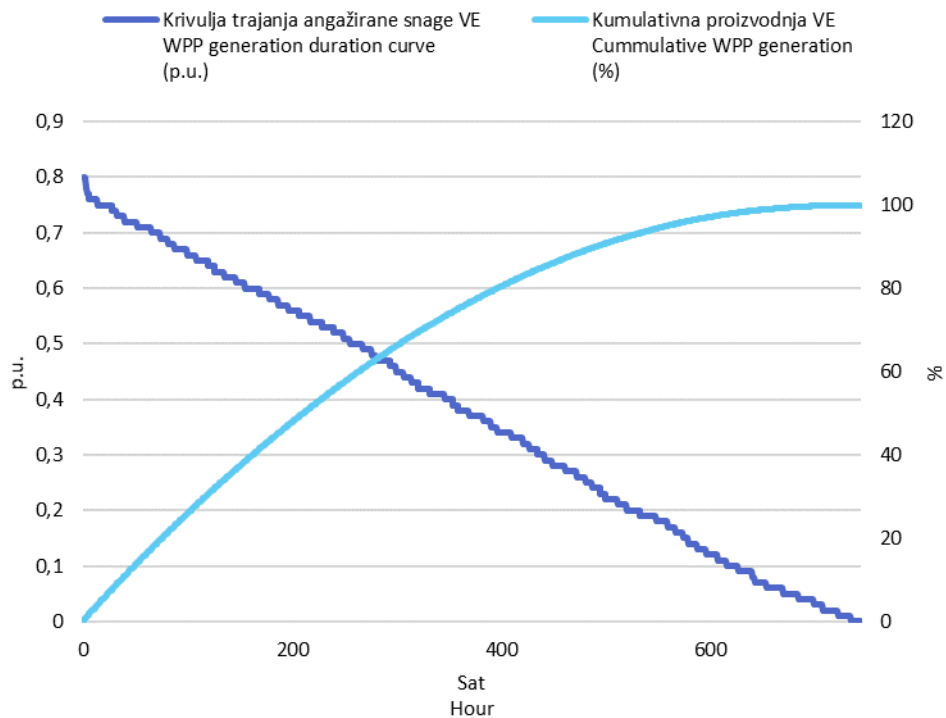
Slika 3 Krivulja trajanja angažirane snage svih VE i kumulativna proizvodnja VE u siječnju 2019. godine u jediničnim vrijednostima
