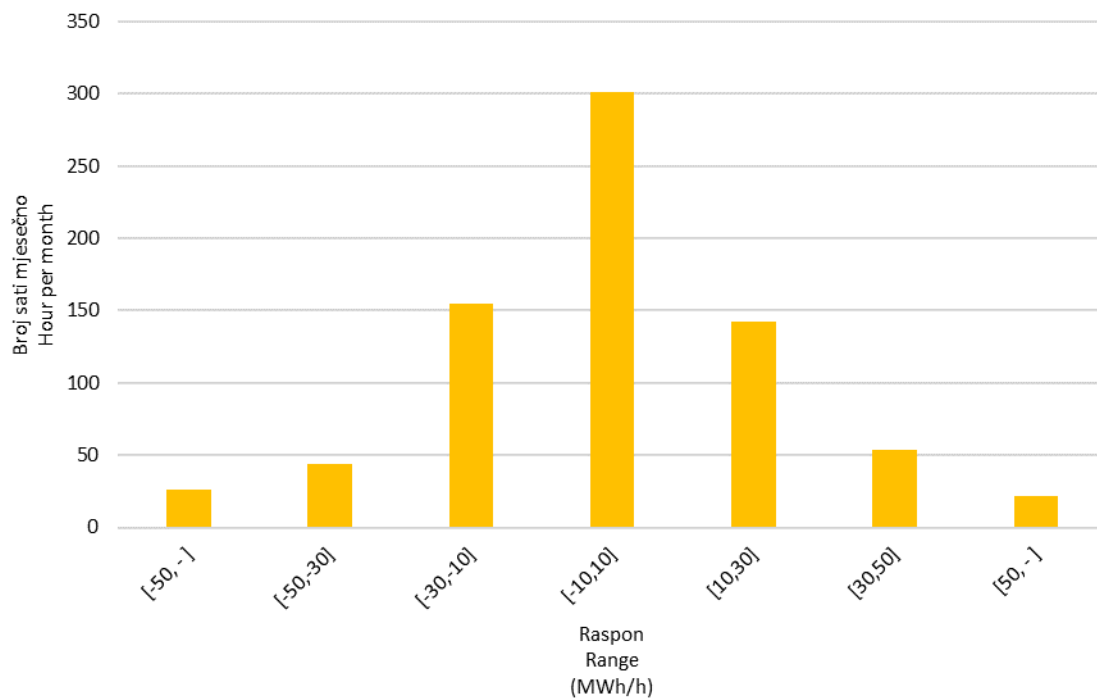
Slika 10 Statistička raspodjela satnih promjena proizvodnje VE u siječnju 2019. godine
