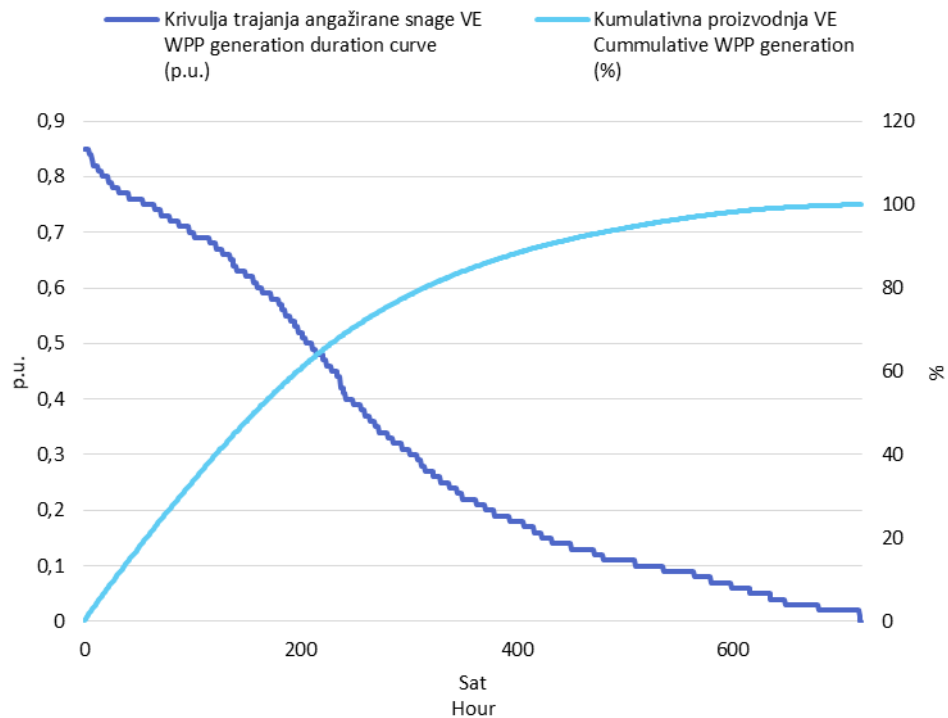
Slika 3 Krivulja trajanja angažirane snage svih VE i kumulativna proizvodnja VE u travnju 2017. godine u jediničnim vrijednostima
