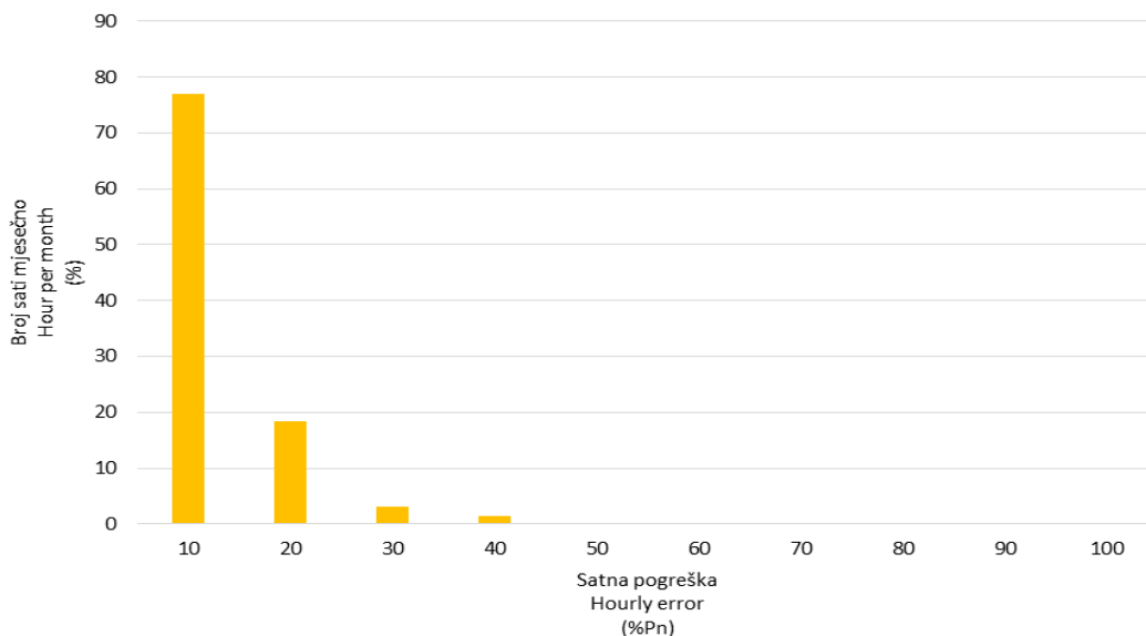
Slika 17 Frekvencija pojavljivanja pogreške prognoze satne proizvodnje svih VE u travnju 2017. godine
