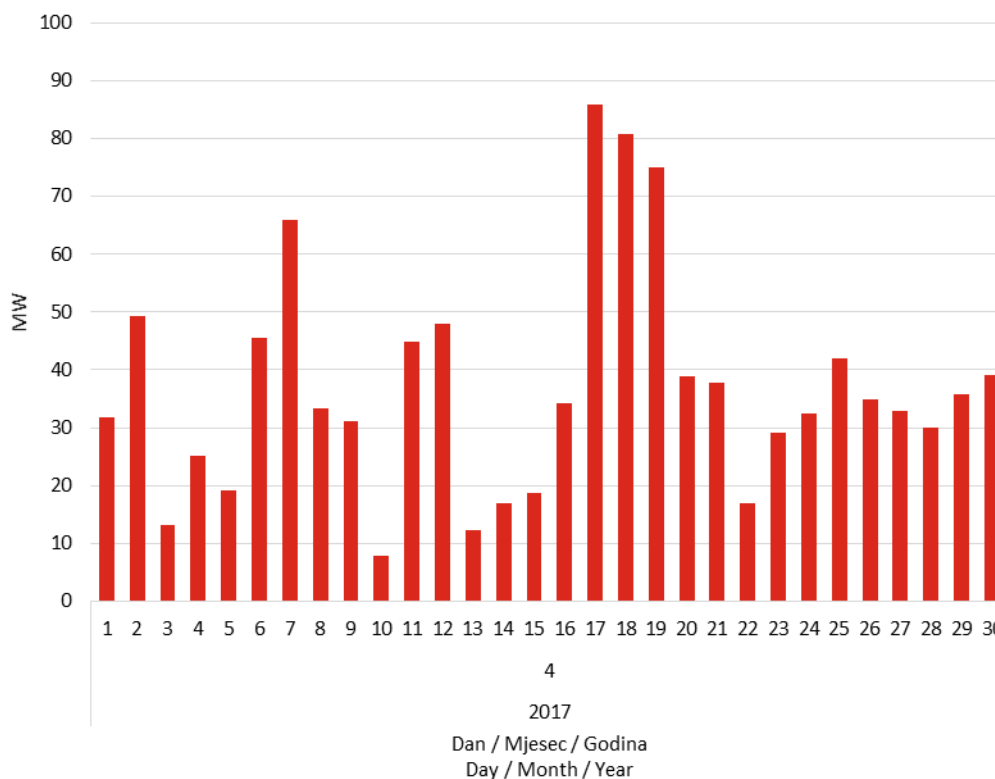
Slika 15 Korijen srednje kvadratne pogreške prognoze satne proizvodnje svih VE u travnju 2017. godine
