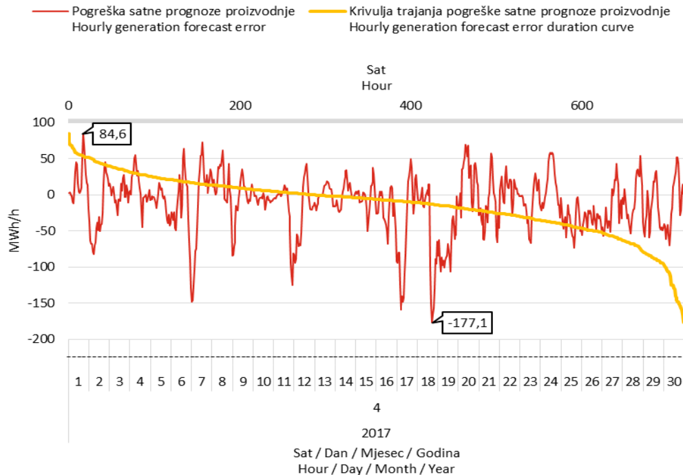
Slika 12 Razlika između prognozirane i ostvarene satne proizvodnje svih VE (pogreška prognoze) i pripadna krivulja trajanja u travnju 2017. godine
