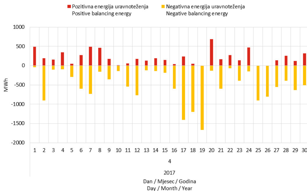
Slika 14 Suma pozitivnih pogreški prognoze satne proizvodnje VE (negativna energija uravnoteženja) i suma negativnih pogreški prognoze satne proizvodnje VE (pozitivna energija uravnoteženja) u travnju 2017. godine
