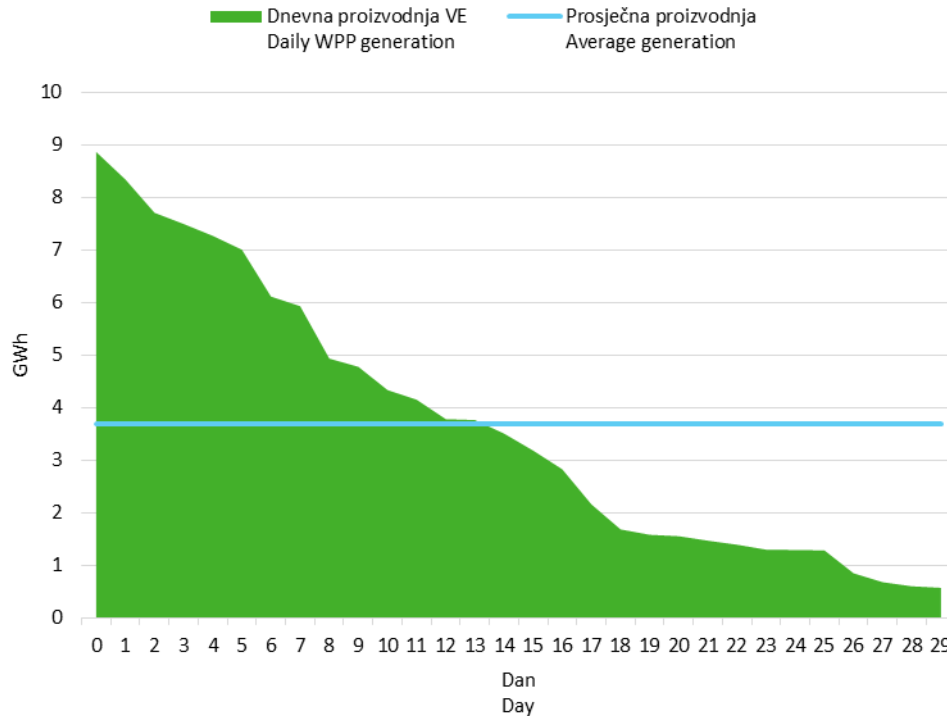
Slika 6 Krivulja trajanja dnevne proizvodnje vjetroelektrana u travnju 2017. godine
