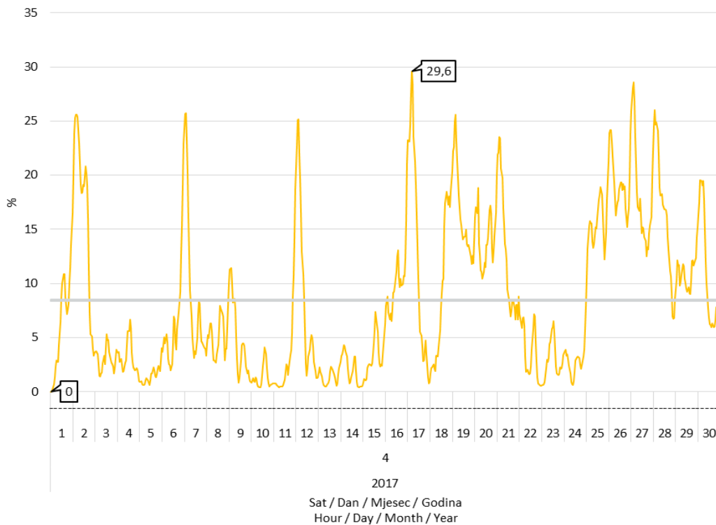
Slika 8 Udio proizvodnje vjetroelektrana u pokrivanju satnog opterećenja elektroenergetskog sustava u travnju 2017. godine
