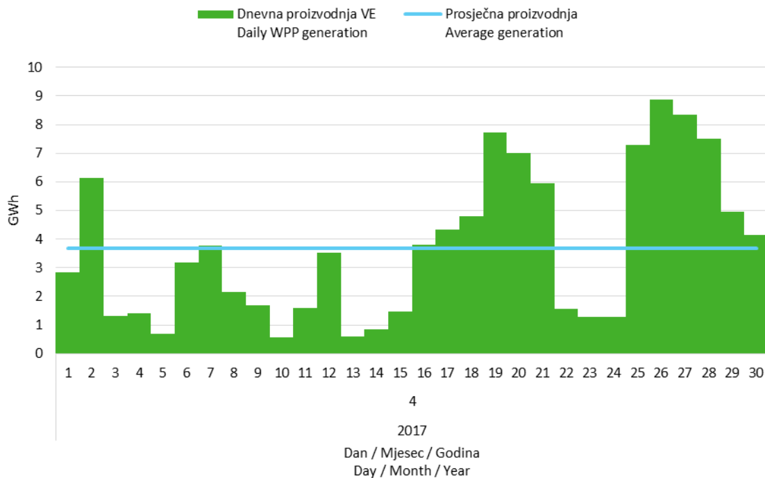
Slika 5 Dnevna proizvodnja svih vjetroelektrana u travnju 2017. godine
