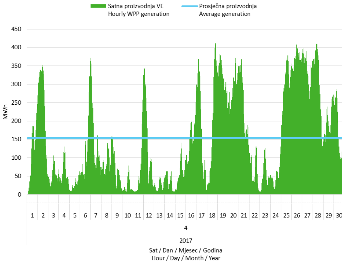
Slika 2 Satna proizvodnja svih vjetroelektrana u travnju 2017. godine
