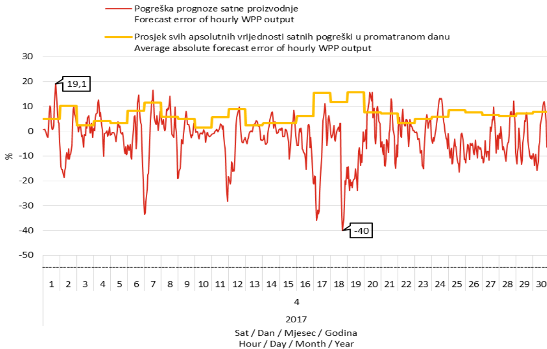
Slika 13 Pogreške prognoze satne proizvodnje VE i prosječne apsolutne pogreške prognoze satne proizvodnje VE na dnevnoj razini iskazane u postocima instalirane snage VE
