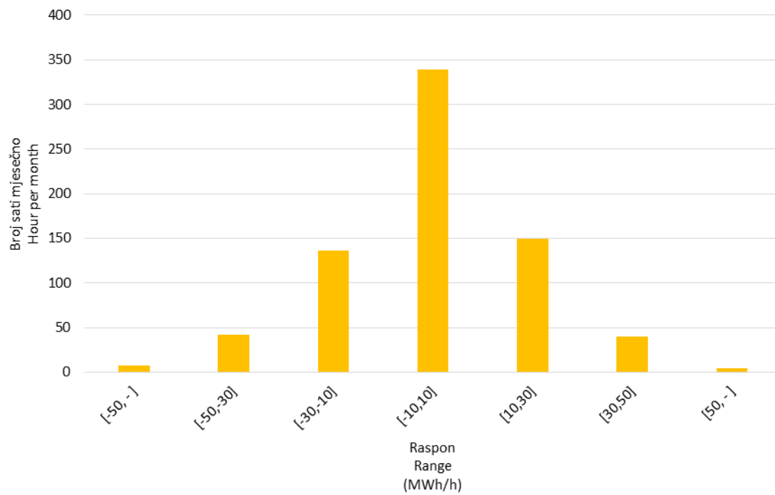
Slika 10 Statistička raspodjela satnih promjena proizvodnje VE u travnju 2017. godine
