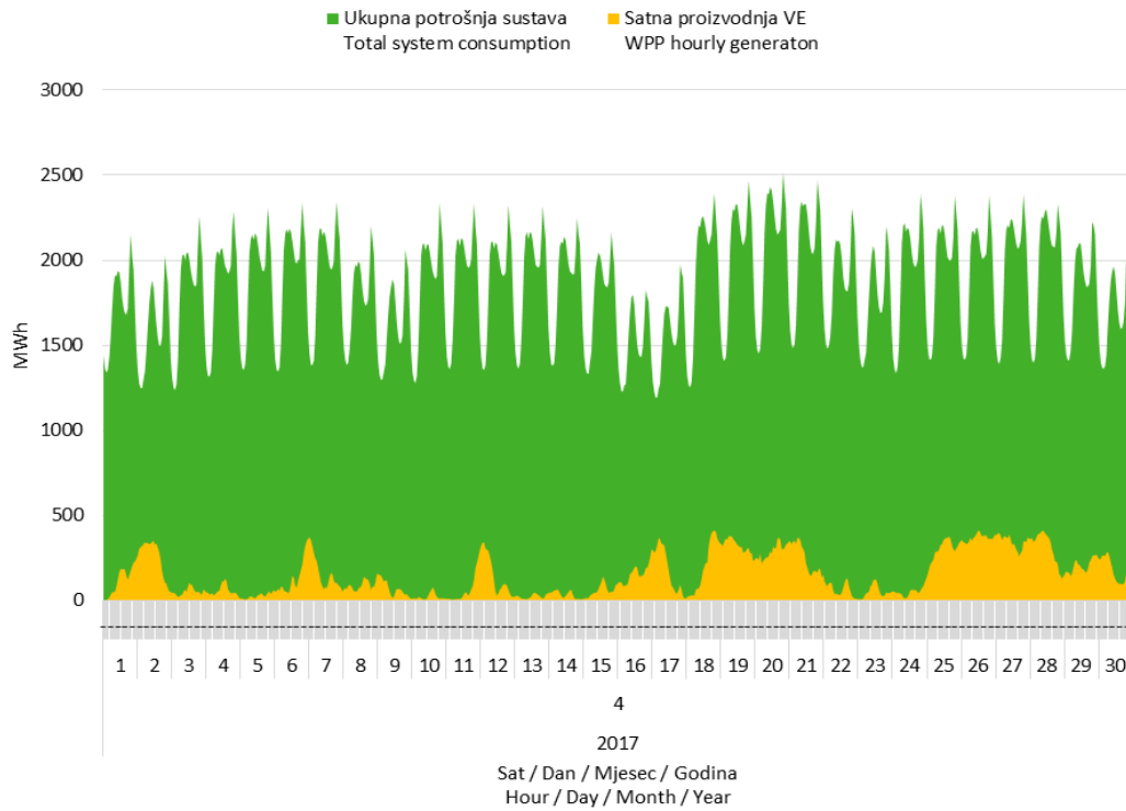
Slika 7 Usporedba satnog dijagrama opterećenja sustava i proizvodnje vjetroelektrana u travnju 2017. godine
