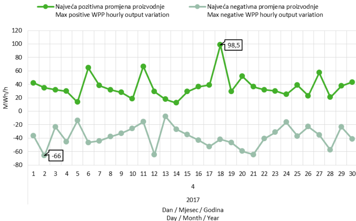
Slika 9 Maksimalna pozitivna i maksimalna negativna promjena satne proizvodnje VE u travnju 2017. godine
