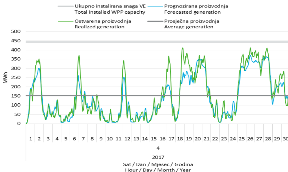
Slika 11 Prognozirana i ostvarena satna proizvodnja vjetroelektrana u travnju 2017. godine
