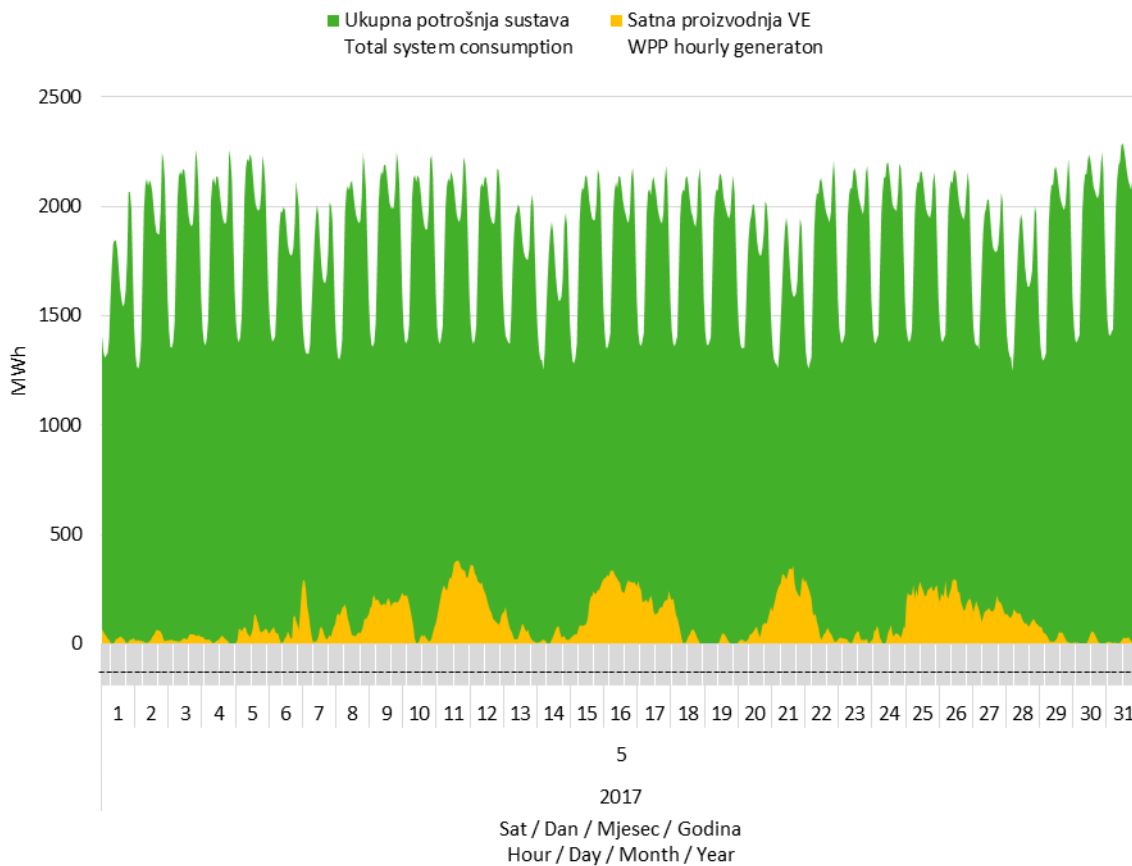
Slika 7 Usporedba satnog dijagrama opterećenja sustava i proizvodnje vjetroelektrana u svibnju 2017. godine
