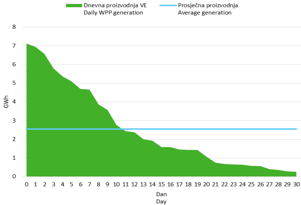
Slika 6 Krivulja trajanja dnevne proizvodnje vjetroelektrana u svibnju 2017. godine
