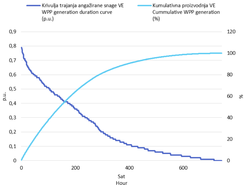
Slika 3 Krivulja trajanja angažirane snage svih VE i kumulativna proizvodnja VE u svibnju 2017. godine u jediničnim vrijednostima
