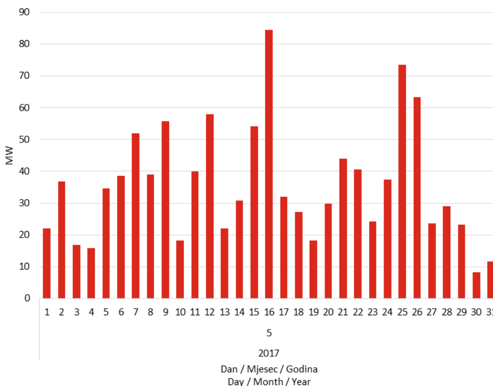
Slika 15 Korijen srednje kvadratne pogreške prognoze satne proizvodnje svih VE u svibnju 2017. godine
