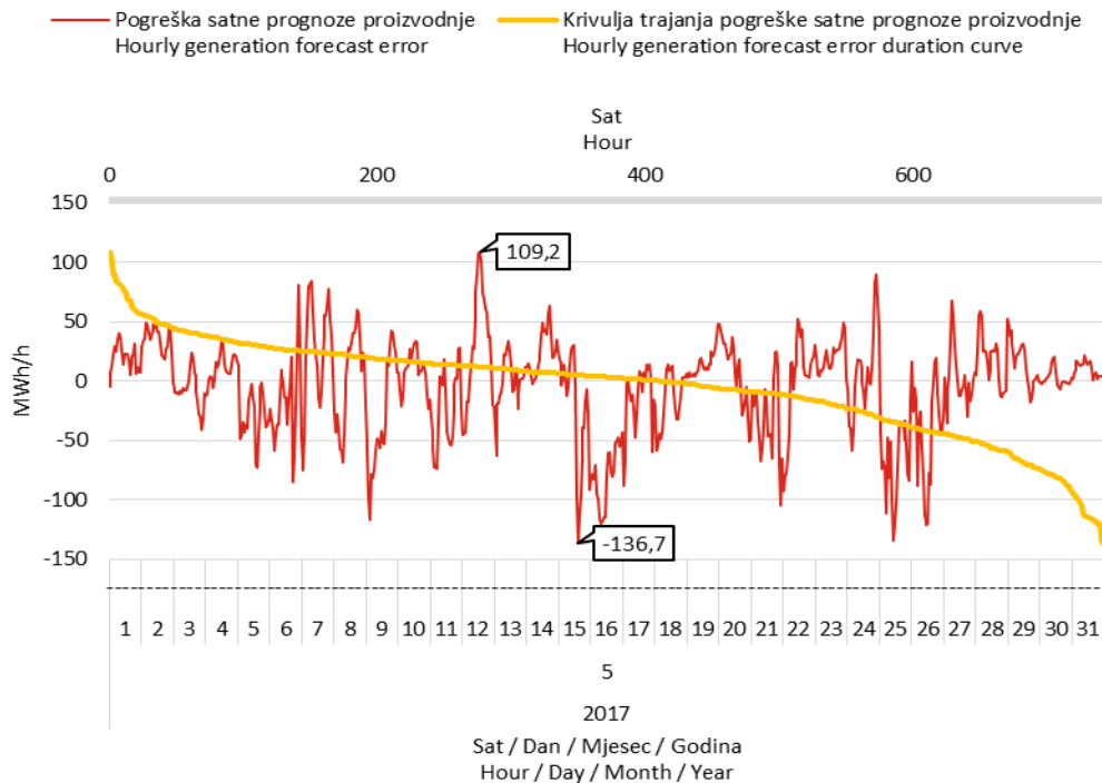
Slika 12 Razlika između prognozirane i ostvarene satne proizvodnje svih VE (pogreška prognoze) i pripadna krivulja trajanja u svibnju 2017. godine
