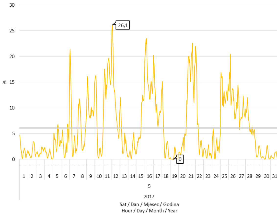
Slika 8 Udio proizvodnje vjetroelektrana u pokrivanju satnog opterećenja elektroenergetskog sustava u svibnju 2017. godine
