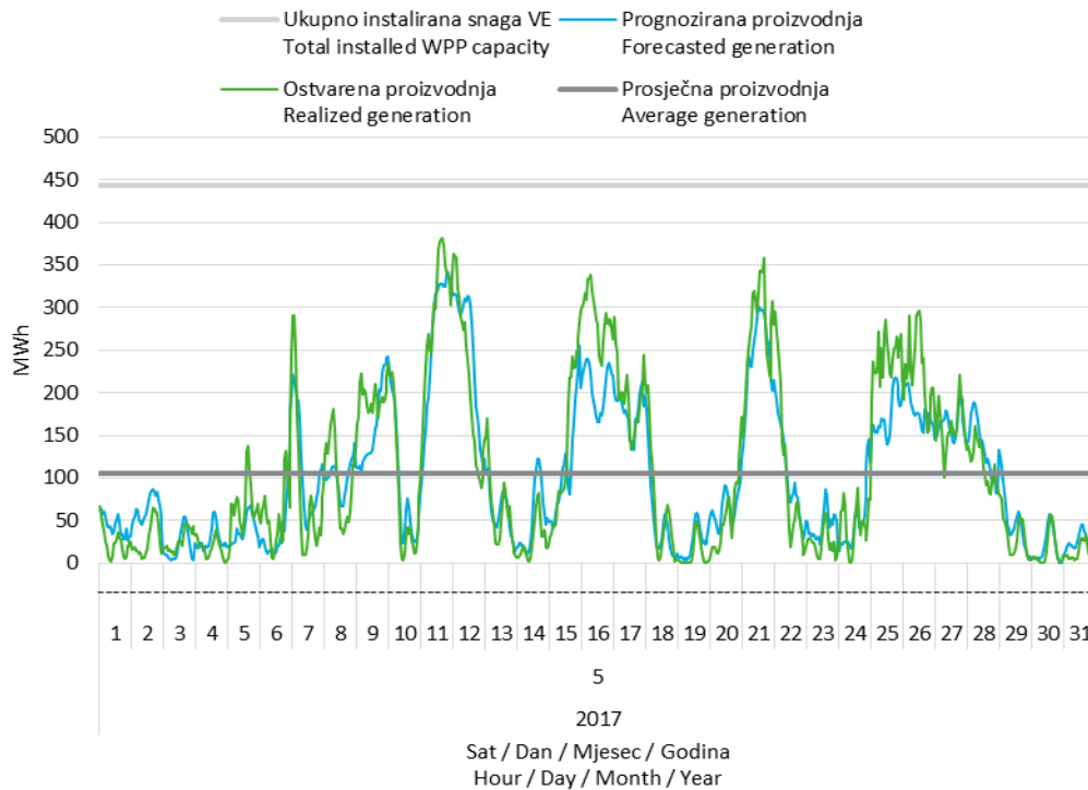
Slika 11 Prognozirana i ostvarena satna proizvodnja vjetroelektrana u svibnju 2017. godine
