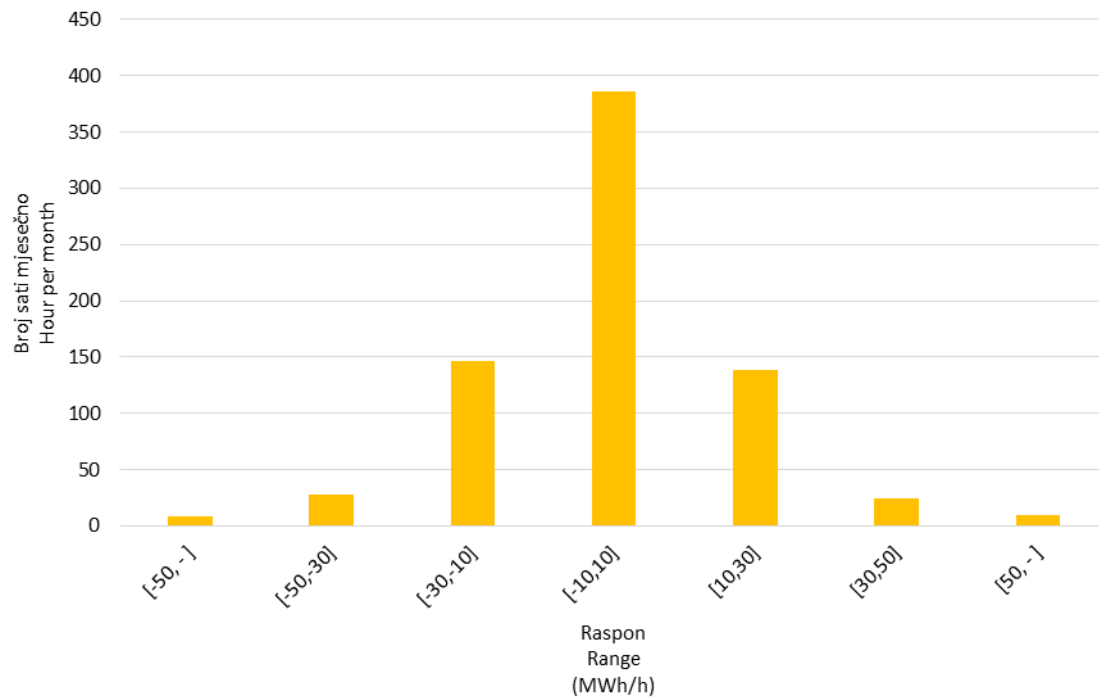
Slika 10 Statistička raspodjela satnih promjena proizvodnje VE u svibnju 2017. godine
