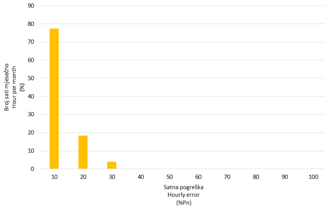
Slika 17 Frekvencija pojavljivanja pogreške prognoze satne proizvodnje svih VE u svibnju 2017. godine
