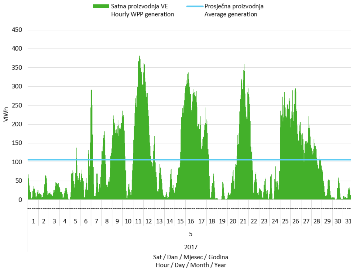
Slika 2 Satna proizvodnja svih vjetroelektrana u svibnju 2017. godine
