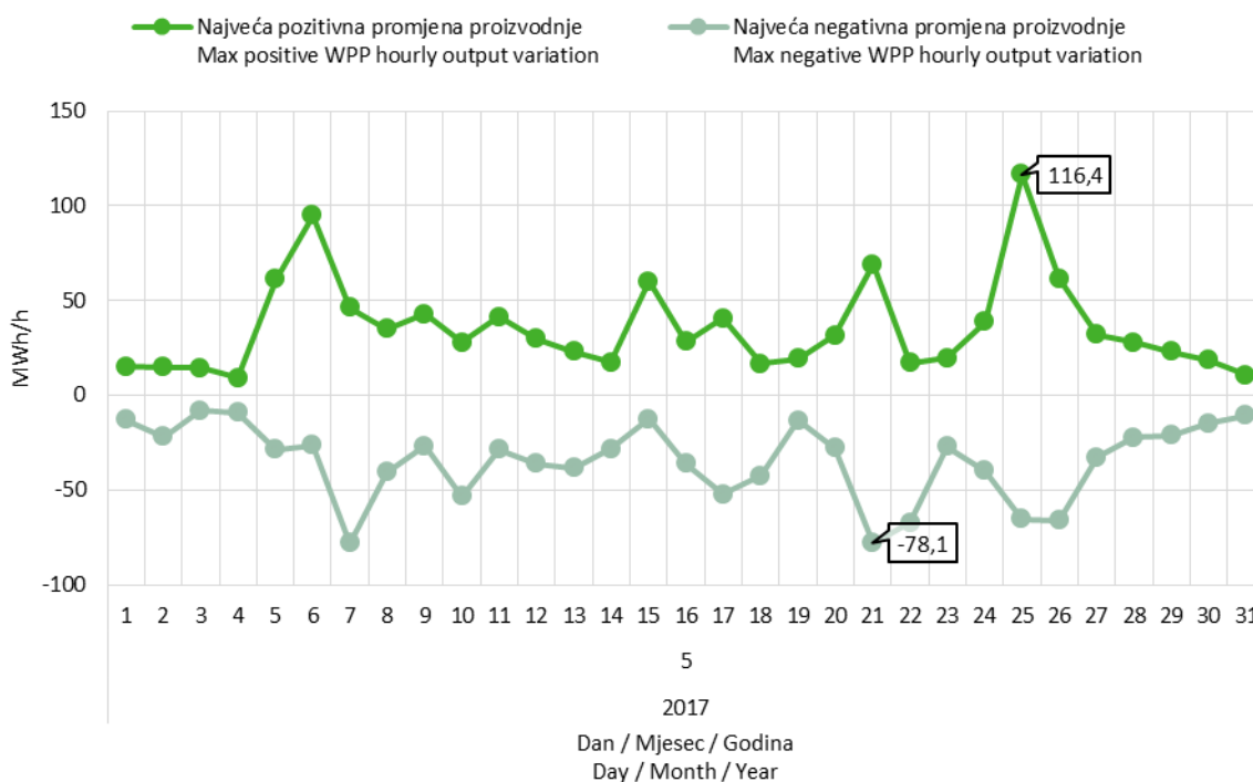
Slika 9 Maksimalna pozitivna i maksimalna negativna promjena satne proizvodnje VE u svibnju 2017. godine
