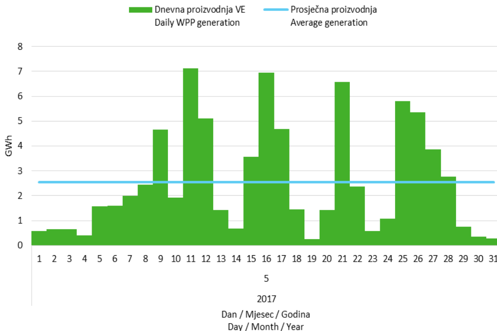
Slika 5 Dnevna proizvodnja svih vjetroelektrana u svibnju 2017. godine Figure 5 Daily generation of all wind power plants in May 2017
