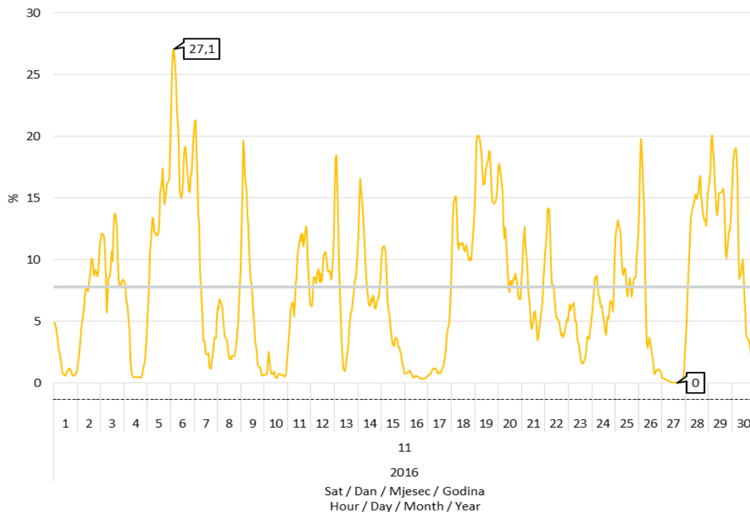
Slika 8 Udio proizvodnje vjetroelektrana u pokrivanju satnog opterećenja elektroenergetskog sustava u studenom 2016. godine
