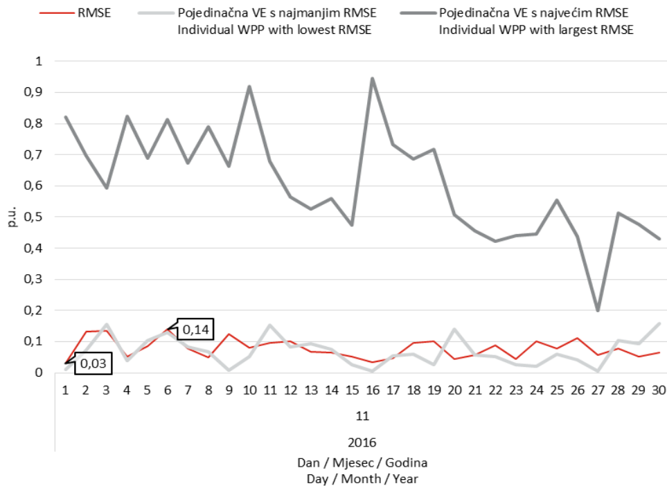
Slika 16 Korijen srednje kvadratne pogreške prognoze satne proizvodnje svih VE u jediničnim vrijednostima
