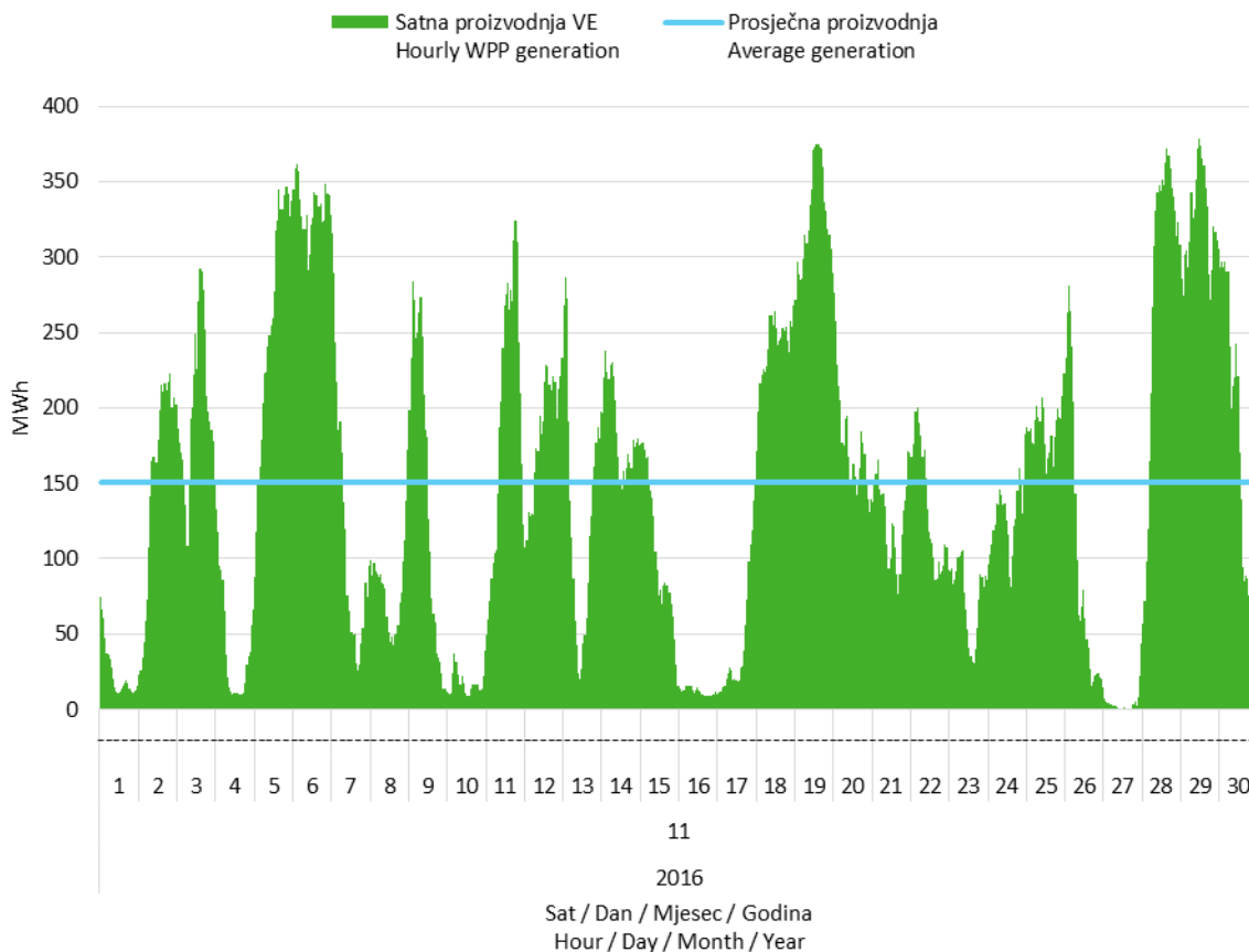
Slika 2 Satna proizvodnja svih vjetroelektrana u studenom 2016. godine
