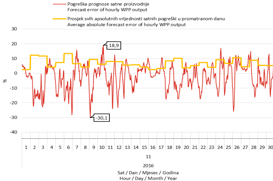
Slika 13 Pogreške prognoze satne proizvodnje VE i prosječne apsolutne pogreške prognoze satne proizvodnje VE na dnevnoj razini iskazane u postocima instalirane snage VE
