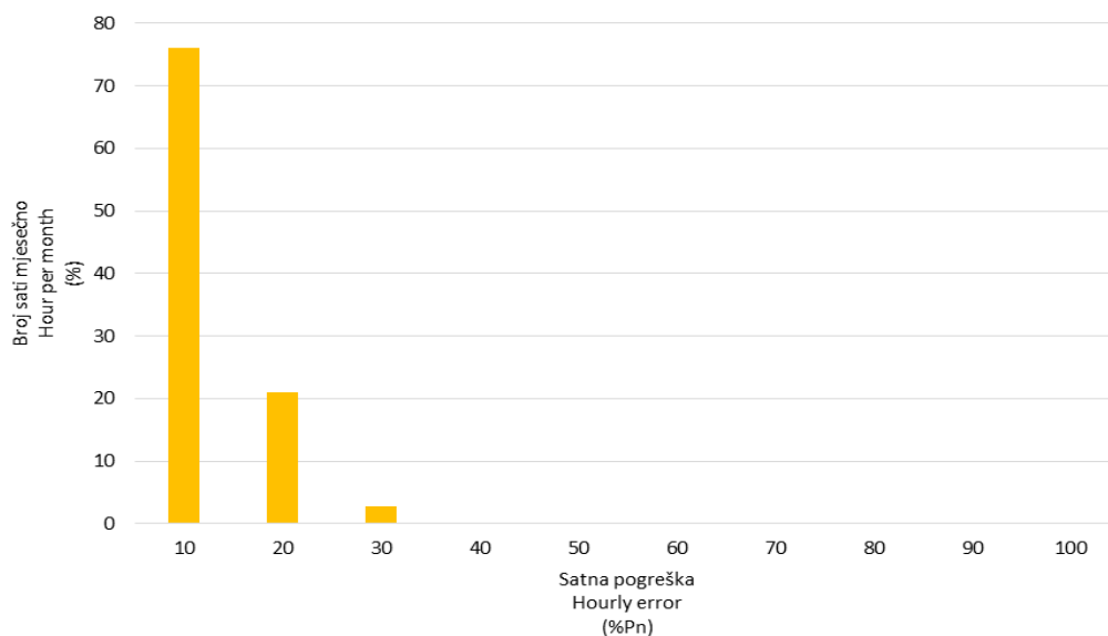
Slika 17 Frekvencija pojavljivanja pogreške prognoze satne proizvodnje svih VE u studenom 2016. godine
