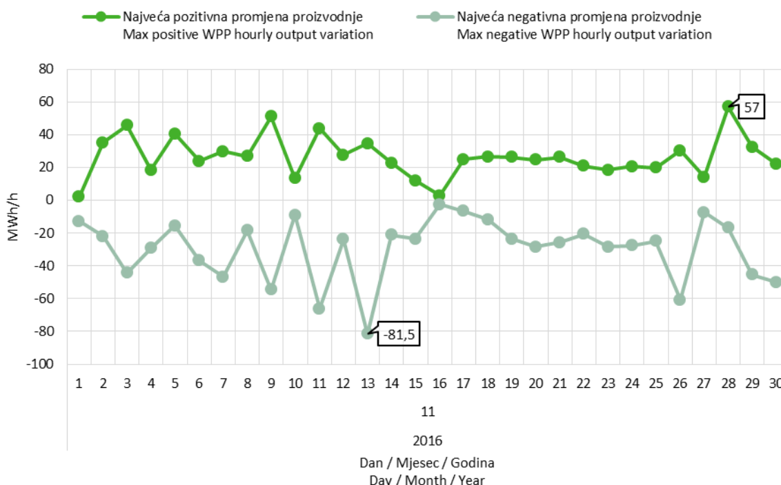
Slika 9 Maksimalna pozitivna i maksimalna negativna promjena satne proizvodnje VE u studenom 2016. godine
