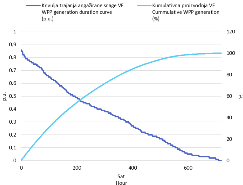
Slika 3 Krivulja trajanja angažirane snage svih VE i kumulativna proizvodnja VE u studenom 2016. godine u jediničnim vrijednostima
