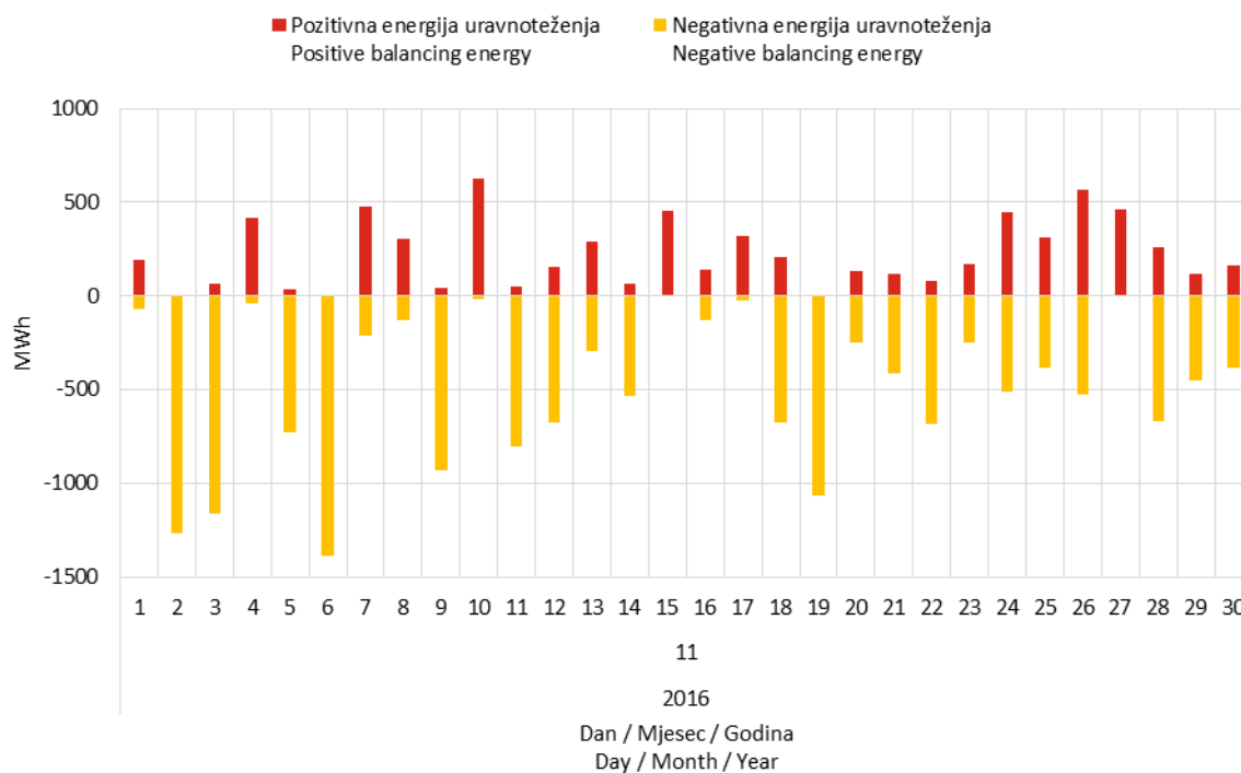
Slika 14 Suma pozitivnih pogreški prognoze satne proizvodnje VE (negativna energija uravnoteženja) i suma negativnih pogreški prognoze satne proizvodnje VE (pozitivna energija uravnoteženja) u studenom 2016. godine
