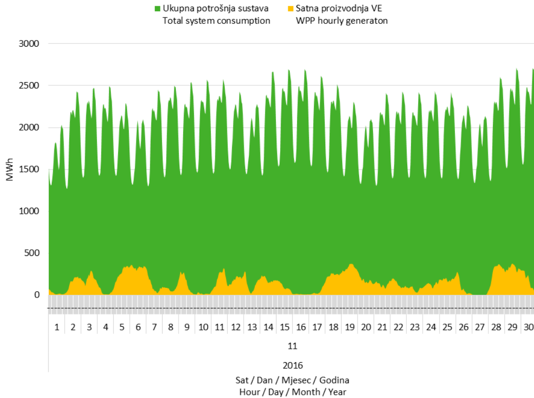
Slika 7 Usporedba satnog dijagrama opterećenja sustava i proizvodnje vjetroelektrana u studenom 2016. godine
