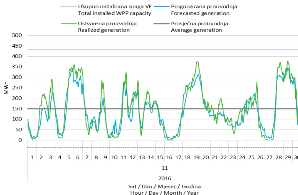
Slika 11 Prognozirana i ostvarena satna proizvodnja vjetroelektrana u studenom 2016. godine
