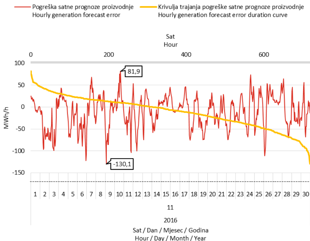
Slika 12 Razlika između prognozirane i ostvarene satne proizvodnje svih VE (pogreška prognoze) i pripadna krivulja trajanja u studenom 2016. godine
