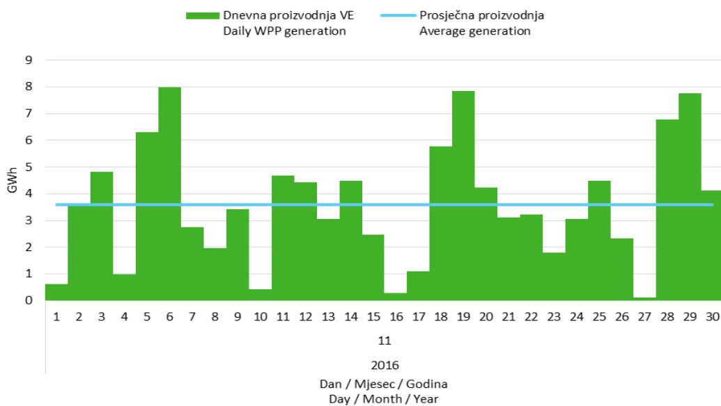
Slika 5 Dnevna proizvodnja svih vjetroelektrana u studenom 2016. godine
