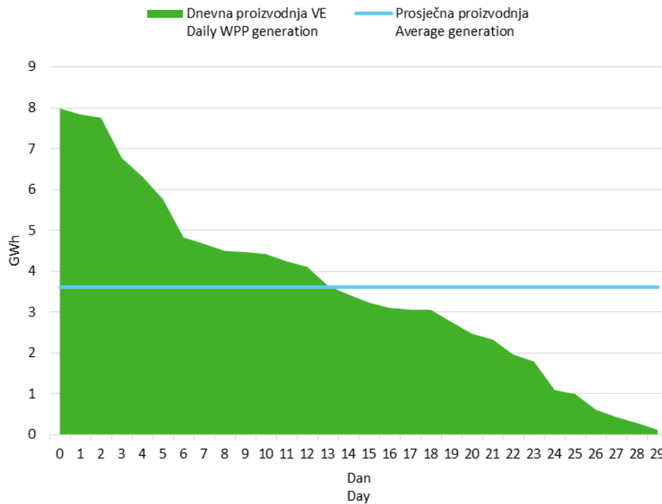
Slika 6 Krivulja trajanja dnevne proizvodnje vjetroelektrana u studenom 2016. godine
