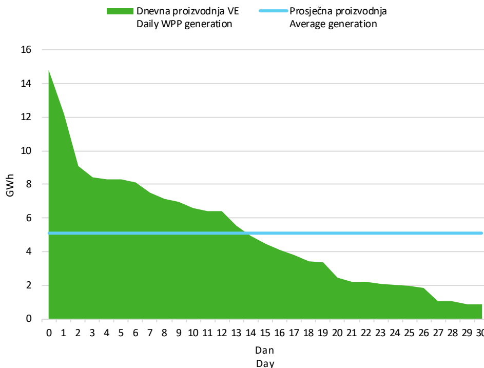
Slika 6 Krivulja trajanja dnevne proizvodnje vjetroelektrana u kolovozu 2024. godine
