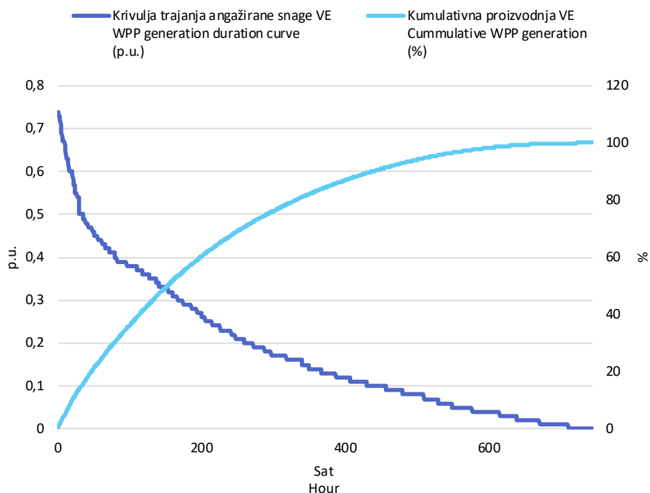
Slika 3 Krivulja trajanja angažirane snage svih VE i kumulativna proizvodnja VE u kolovozu 2024. godine u jediničnim vrijednostima
