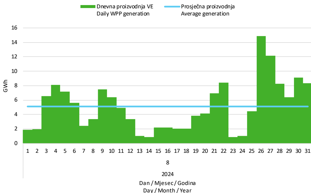
Slika 5 Dnevna proizvodnja svih vjetroelektrana u kolovozu 2024. godine
