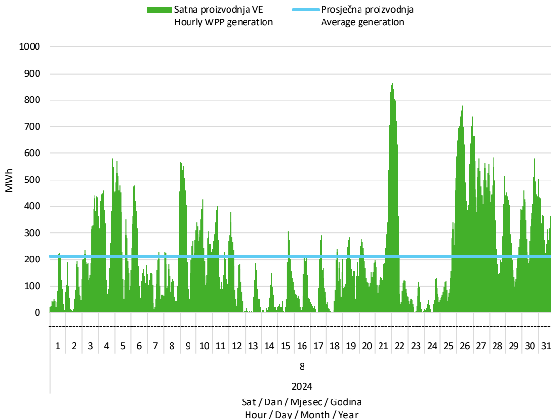
Slika 2 Satna proizvodnja svih vjetroelektrana u kolovozu 2024. godine
