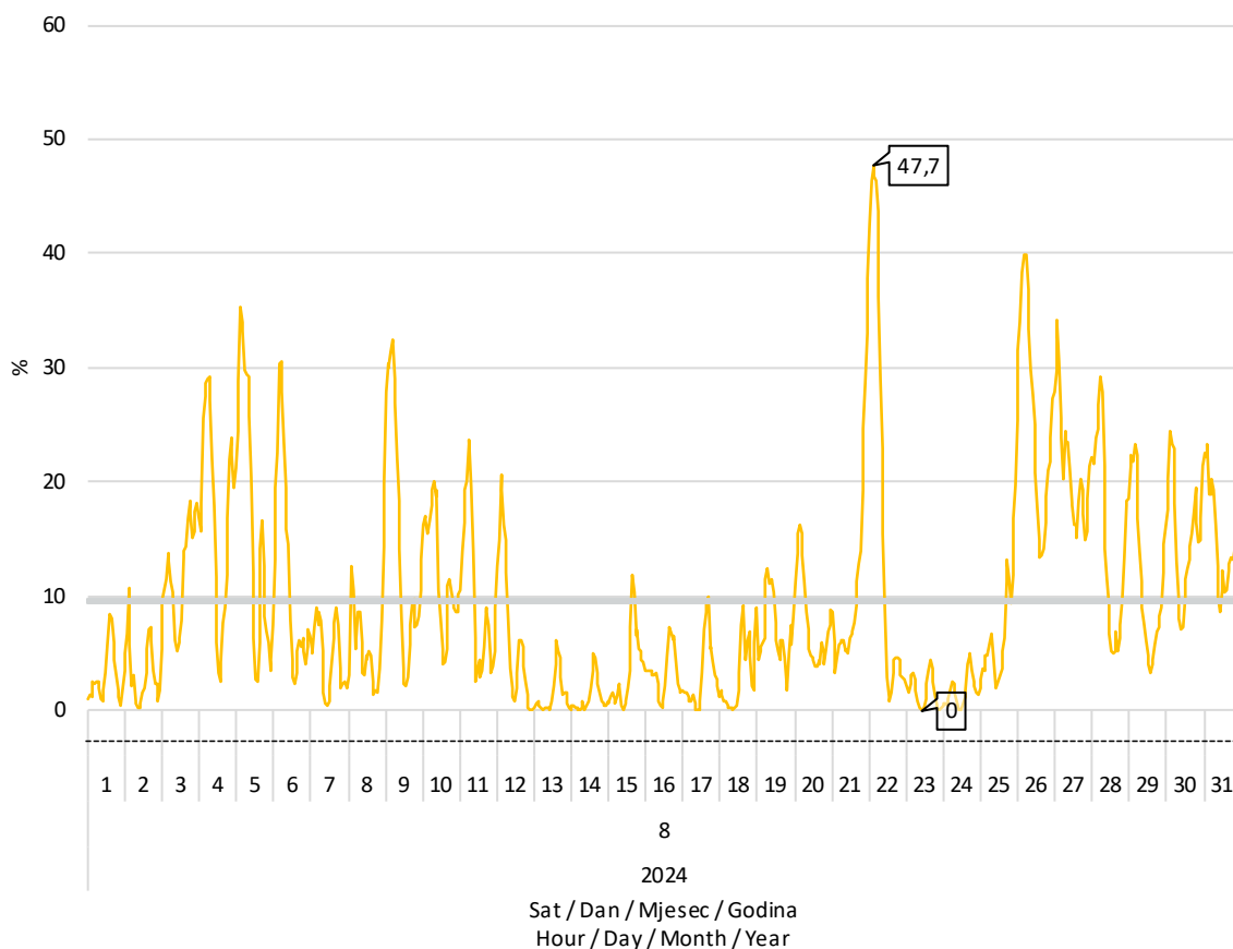
Slika 8 Udio proizvodnje vjetroelektrana u pokrivanju satnog opterećenja elektroenergetskog sustava u kolovozu 2024. godine
