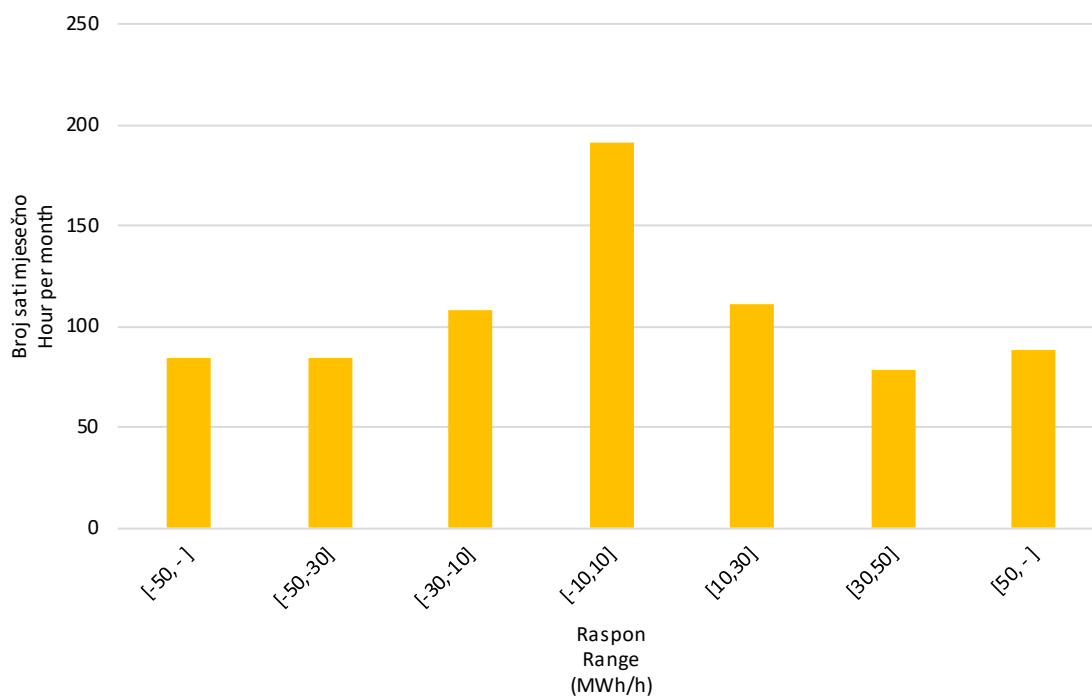
Slika 10 Statistička raspodjela satnih promjena proizvodnje VE u kolovozu 2024. godine
