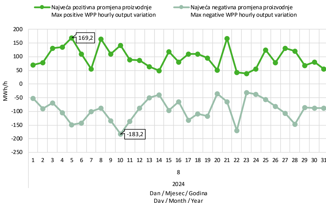
Slika 9 Maksimalna pozitivna i maksimalna negativna promjena satne proizvodnje VE u kolovozu 2024. godine
