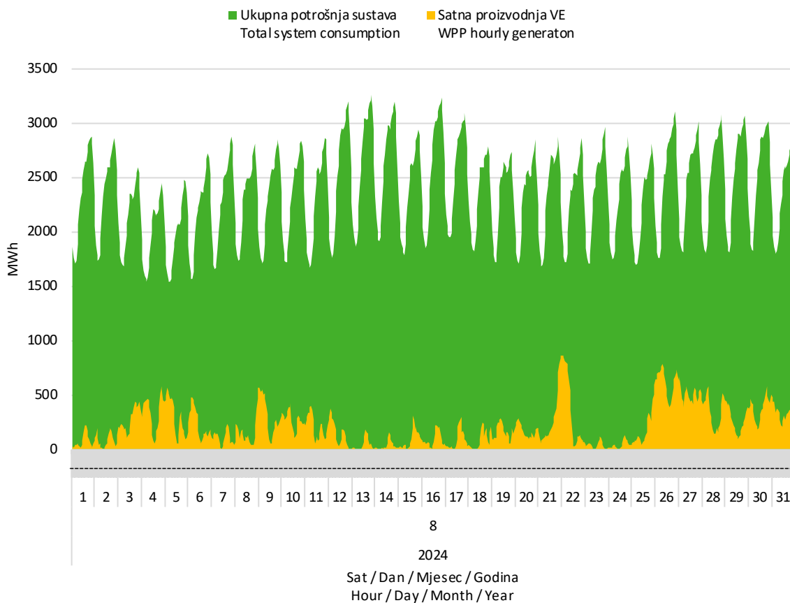
Slika 7 Usporedba satnog dijagrama opterećenja sustava i proizvodnje vjetroelektrana u kolovozu 2024. godine
