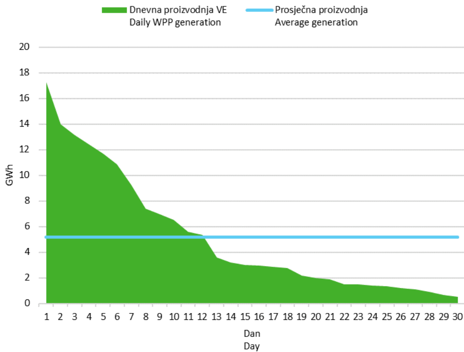
Slika 6 Krivulja trajanja dnevne proizvodnje vjetroelektrana u lipnju 2023. godine
