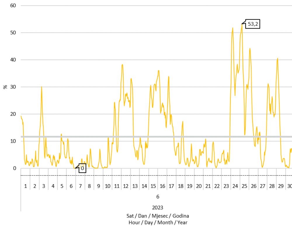
Slika 8 Udio proizvodnje vjetroelektrana u pokrivanju satnog opterećenja elektroenergetskog sustava u lipnju 2023. godine
