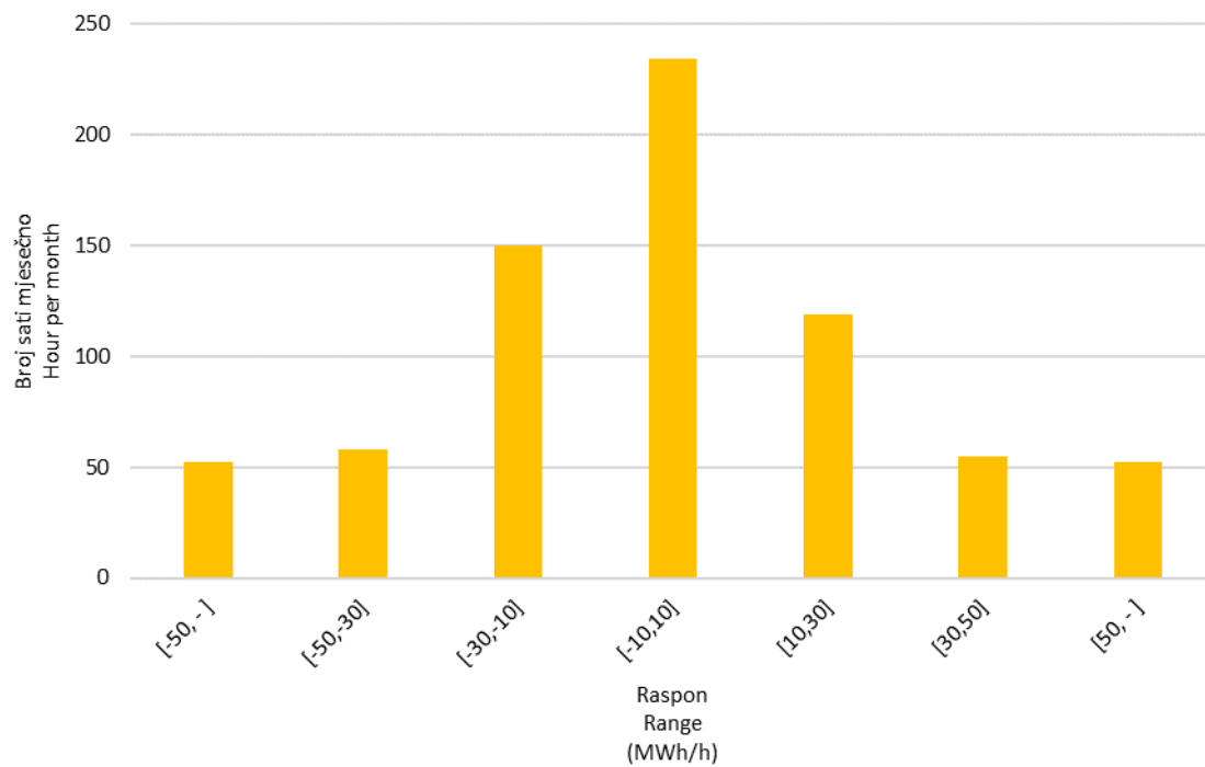
Slika 10 Statistička raspodjela satnih promjena proizvodnje VE u lipnju 2023. godine
