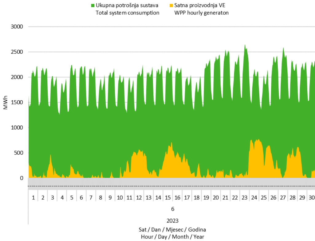
Slika 7 Usporedba satnog dijagrama opterećenja sustava i proizvodnje vjetroelektrana u lipnju 2023. godine
