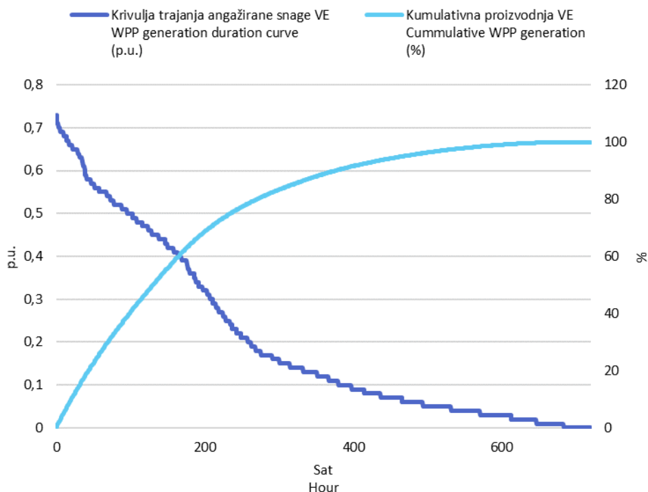
Slika 3 Krivulja trajanja angažirane snage svih VE i kumulativna proizvodnja VE u lipnju 2023. godine u jediničnim vrijednostima
