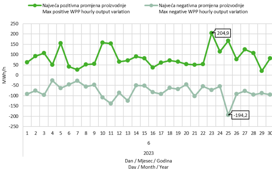
Slika 9 Maksimalna pozitivna i maksimalna negativna promjena satne proizvodnje VE u lipnju 2023. godine
