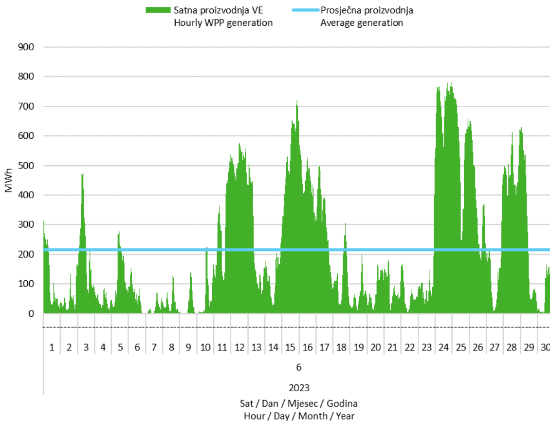
Slika 2 Satna proizvodnja svih vjetroelektrana u lipnju 2023. godine
