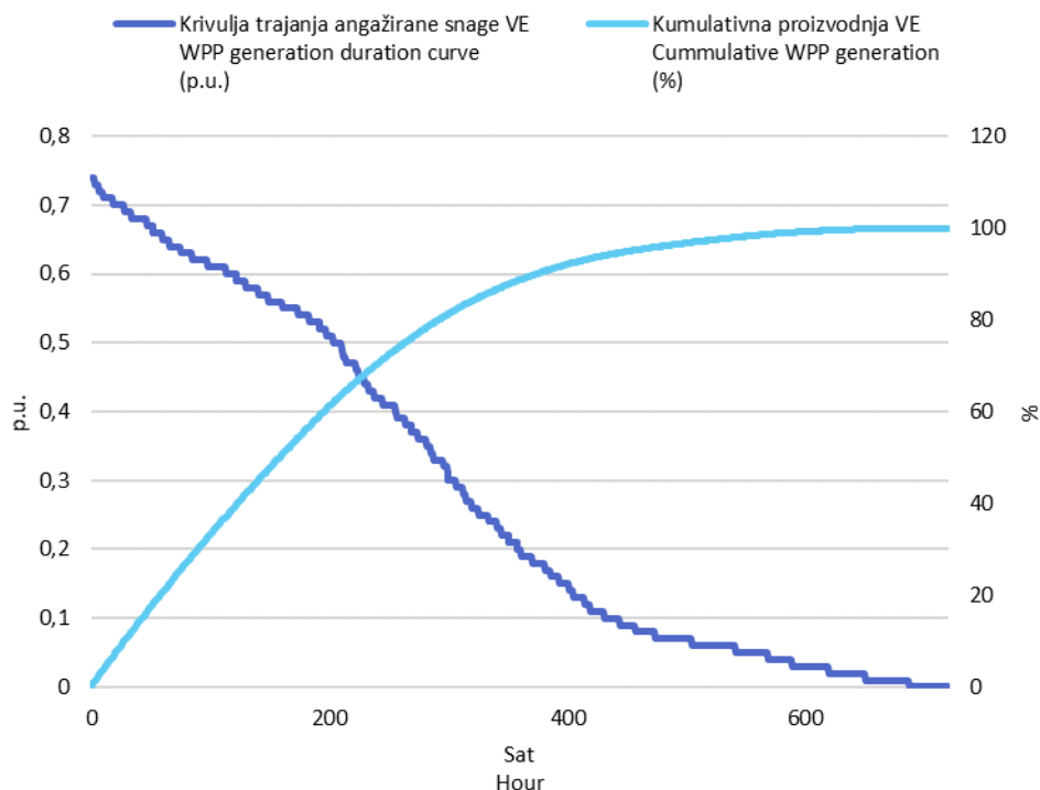
Slika 3 Krivulja trajanja angažirane snage svih VE i kumulativna proizvodnja VE u rujnu 2023. godine u jediničnim vrijednostima
