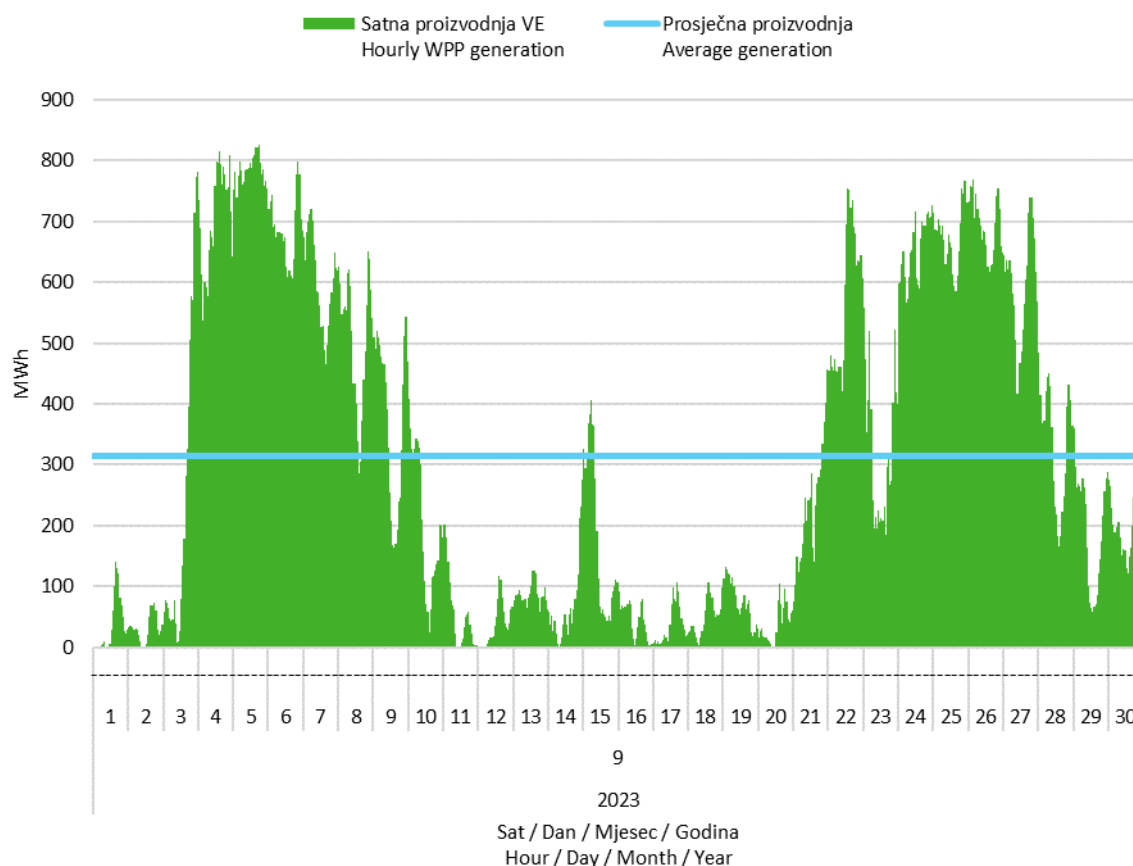
Slika 2 Satna proizvodnja svih vjetroelektrana u rujnu 2023. godine
