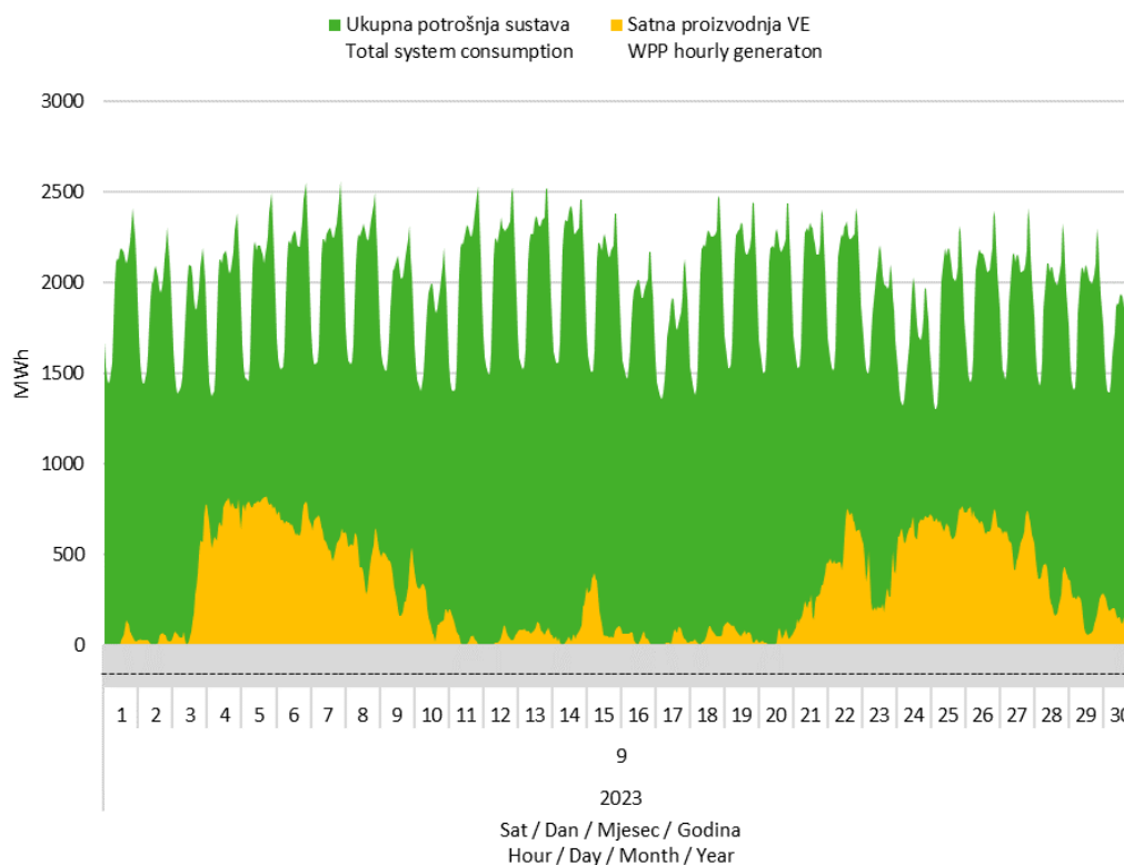
Slika 7 Usporedba satnog dijagrama opterećenja sustava i proizvodnje vjetroelektrana u rujnu 2023. godine
