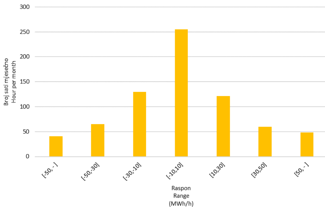
Slika 10 Statistička raspodjela satnih promjena proizvodnje VE u rujnu 2023. godine
