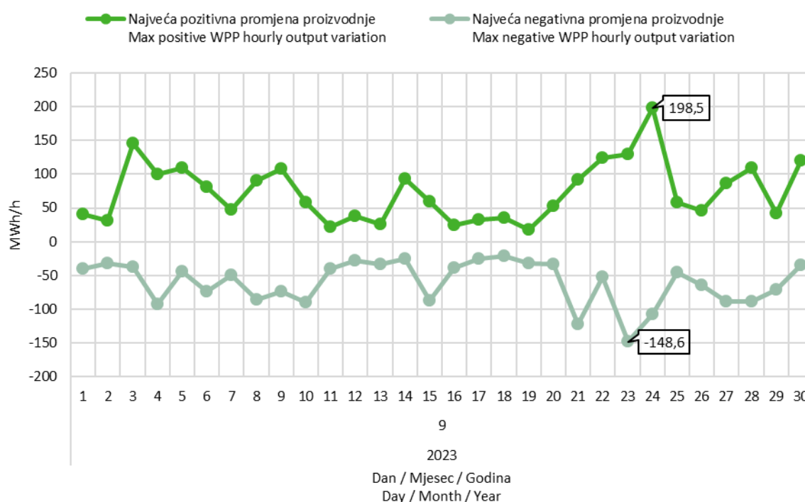
Slika 9 Maksimalna pozitivna i maksimalna negativna promjena satne proizvodnje VE u rujnu 2023. godine
