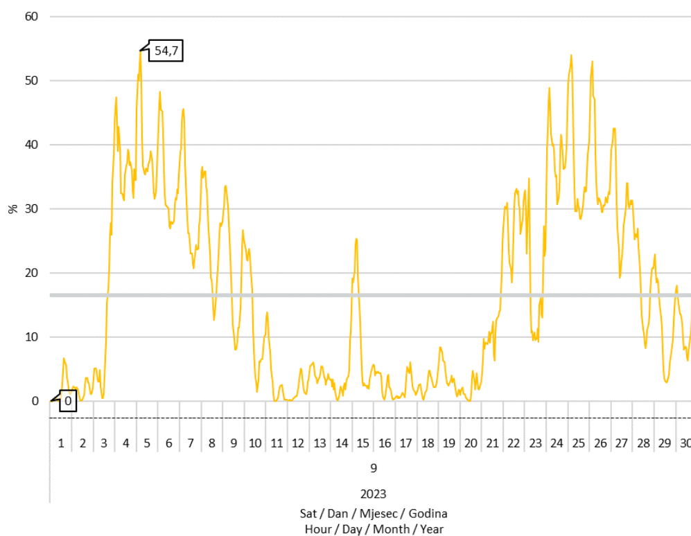
Slika 8 Udio proizvodnje vjetroelektrana u pokrivanju satnog opterećenja elektroenergetskog sustava u rujnu 2023. godine
