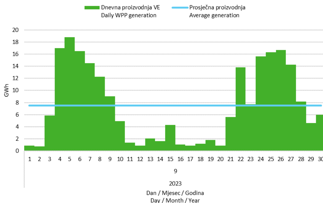
Slika 5 Dnevna proizvodnja svih vjetroelektrana u rujnu 2023. godine
