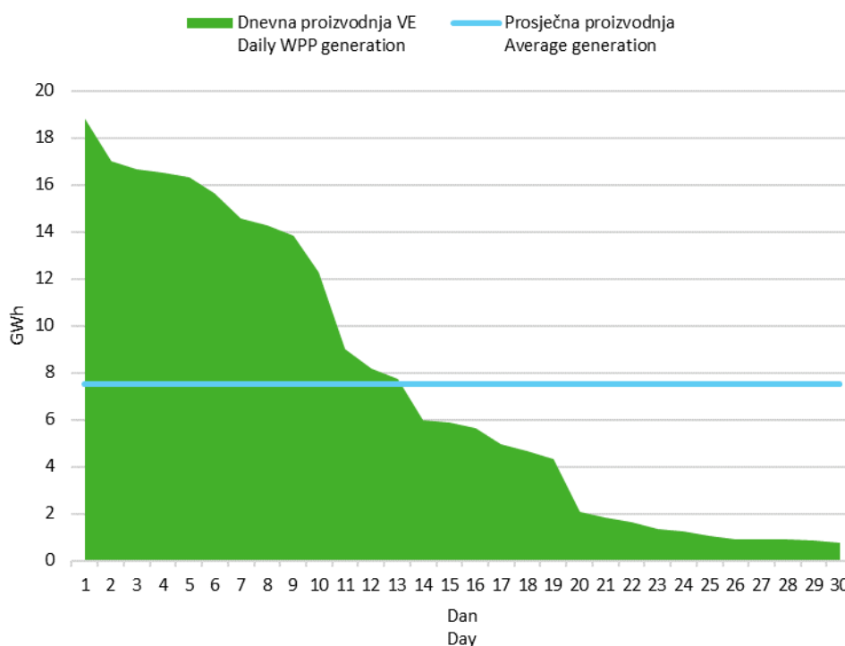
Slika 6 Krivulja trajanja dnevne proizvodnje vjetroelektrana u rujnu 2023. godine
