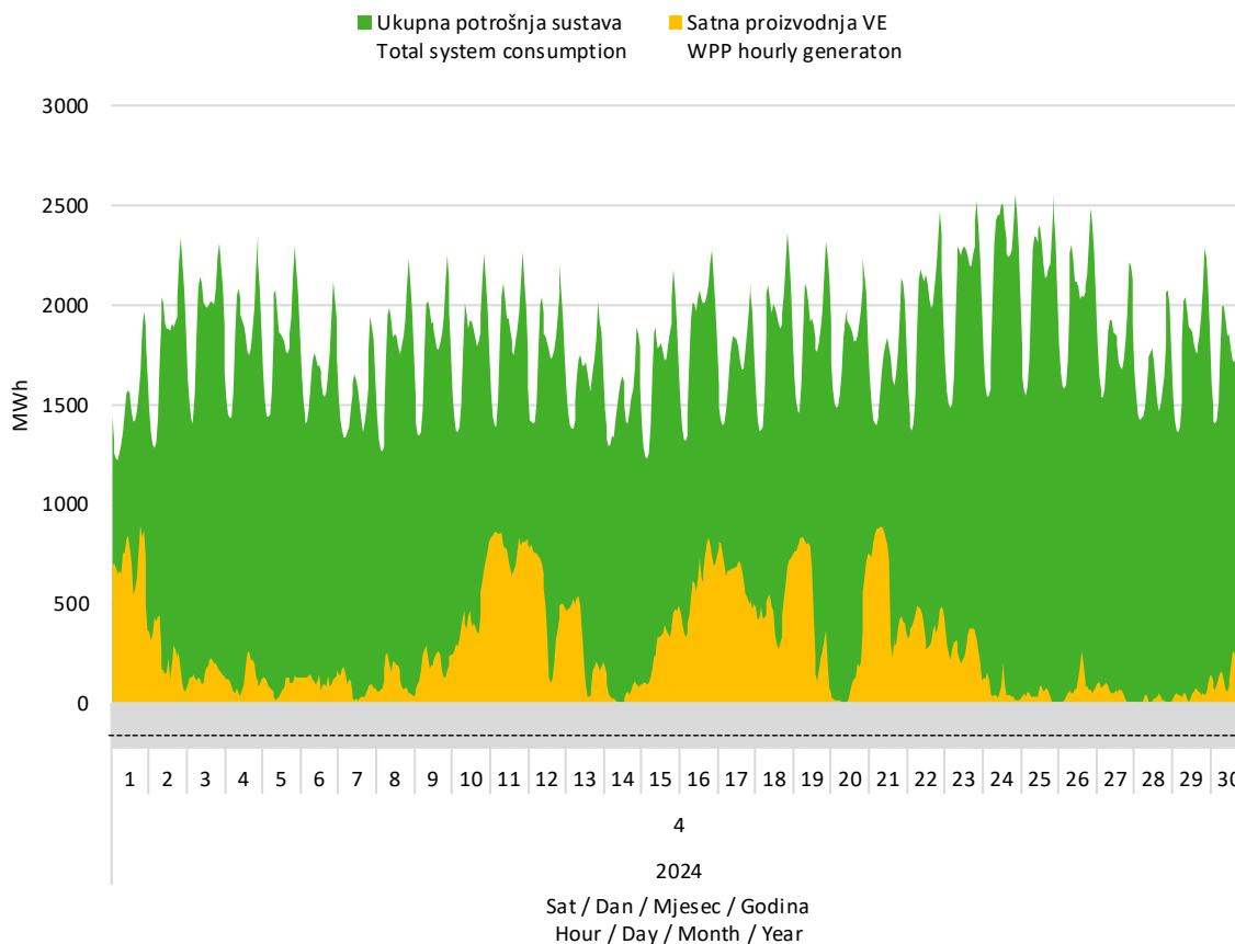
Slika 7 Usporedba satnog dijagrama opterećenja sustava i proizvodnje vjetroelektrana u travnju 2024. godine
