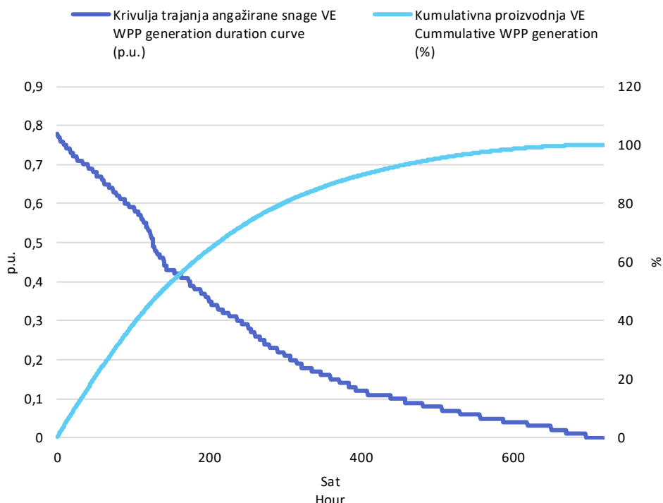
Slika 3 Krivulja trajanja angažirane snage svih VE i kumulativna proizvodnja VE u travnju 2024. godine u jediničnim vrijednostima
