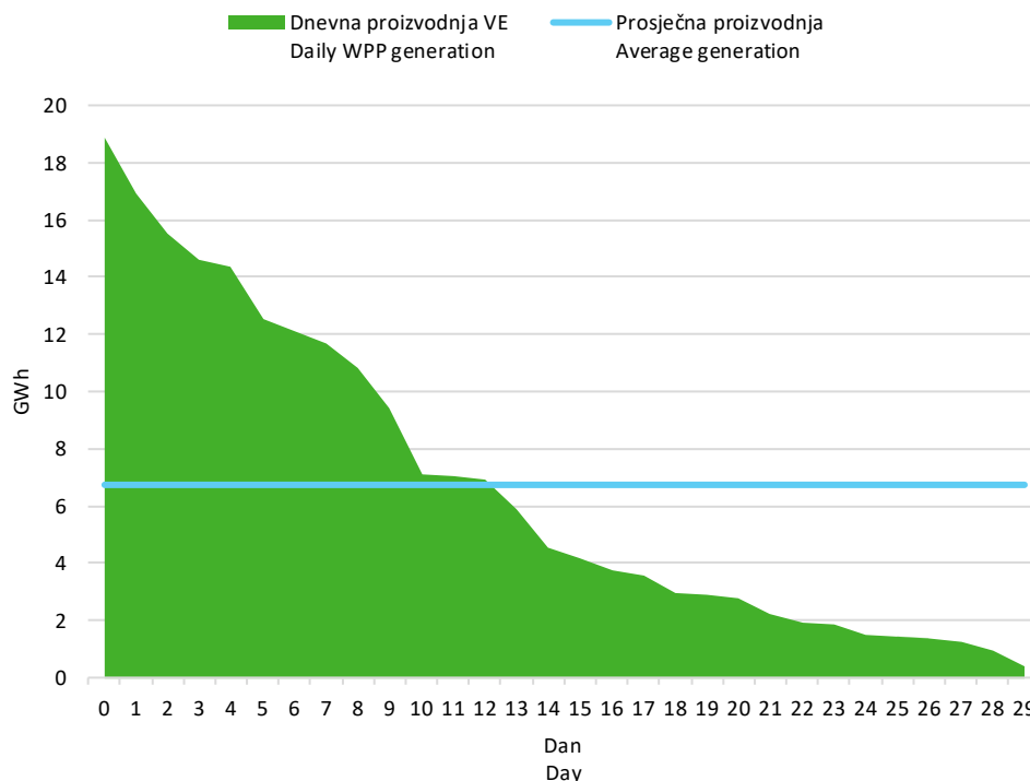
Slika 6 Krivulja trajanja dnevne proizvodnje vjetroelektrana u travnju 2024. godine
