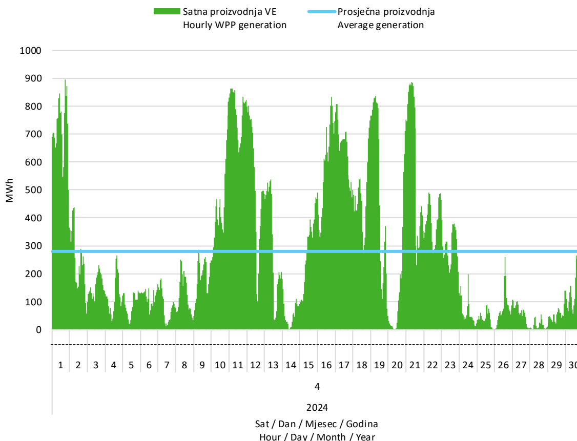
Slika 2 Satna proizvodnja svih vjetroelektrana u travnju 2024. godine
