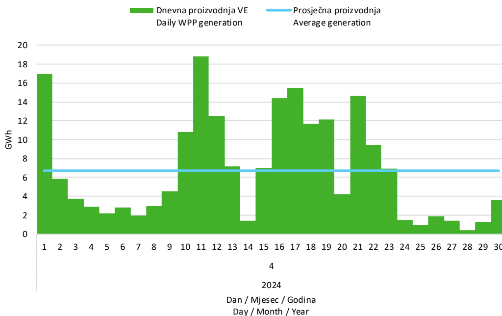
Slika 5 Dnevna proizvodnja svih vjetroelektrana u travnju 2024. godine Figure 5 Daily generation of all wind power plants in April 2024
