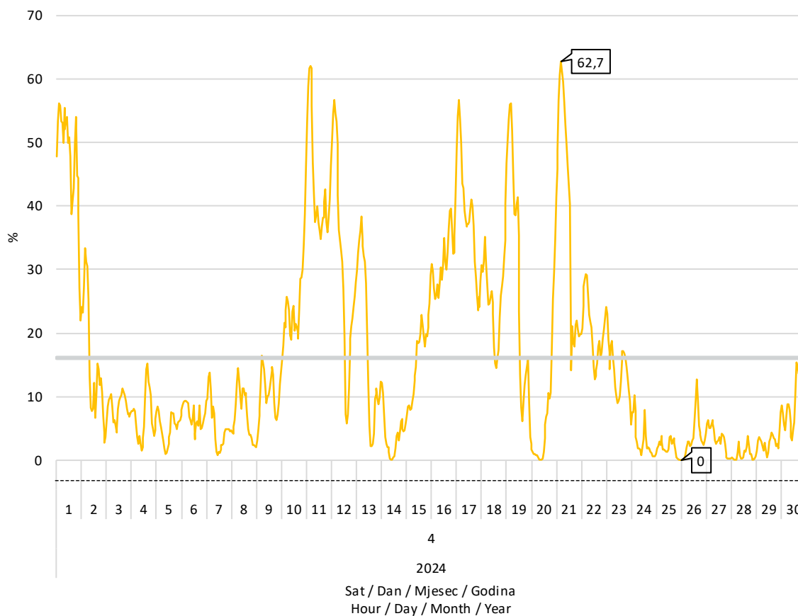
Slika 8 Udio proizvodnje vjetroelektrana u pokrivanju satnog opterećenja elektroenergetskog sustava u travnju 2024. godine
