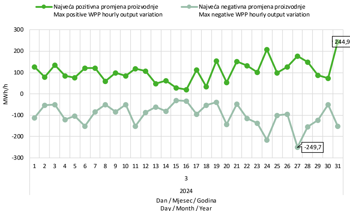
Slika 9 Maksimalna pozitivna i maksimalna negativna promjena satne proizvodnje VE u ožujku 2024. godine
