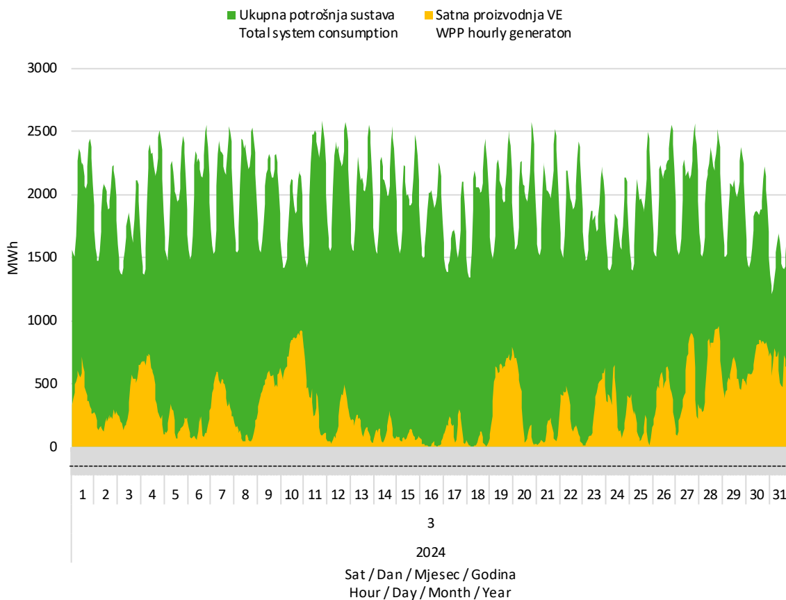
Slika 7 Usporedba satnog dijagrama opterećenja sustava i proizvodnje vjetroelektrana u ožujku 2024. godine
