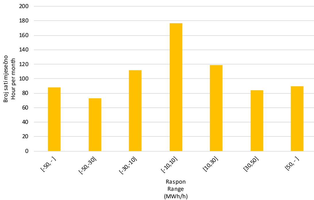
Slika 10 Statistička raspodjela satnih promjena proizvodnje VE u ožujku 2024. godine Figure 10 Statistical distribution of WPP hourly output variations in March 2024
