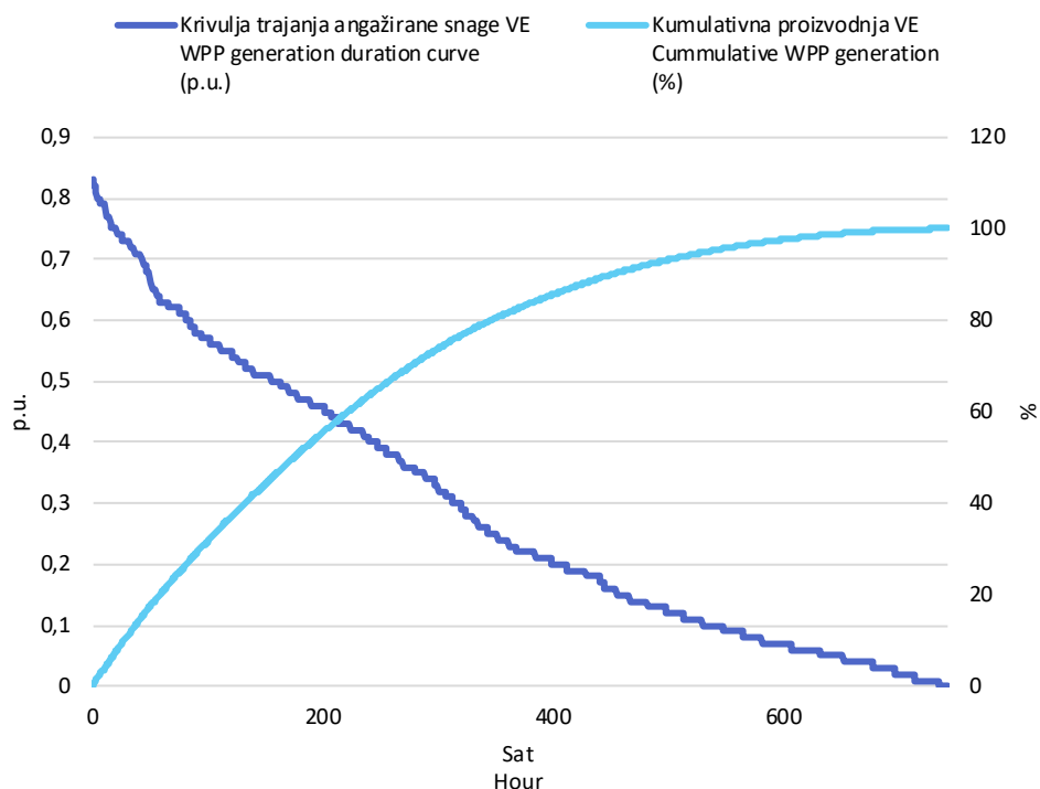
Slika 3 Krivulja trajanja angažirane snage svih VE i kumulativna proizvodnja VE u ožujku 2024. godine u jediničnim vrijednostima
