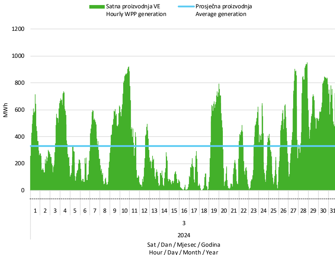
Slika 2 Satna proizvodnja svih vjetroelektrana u ožujku 2024. godine
