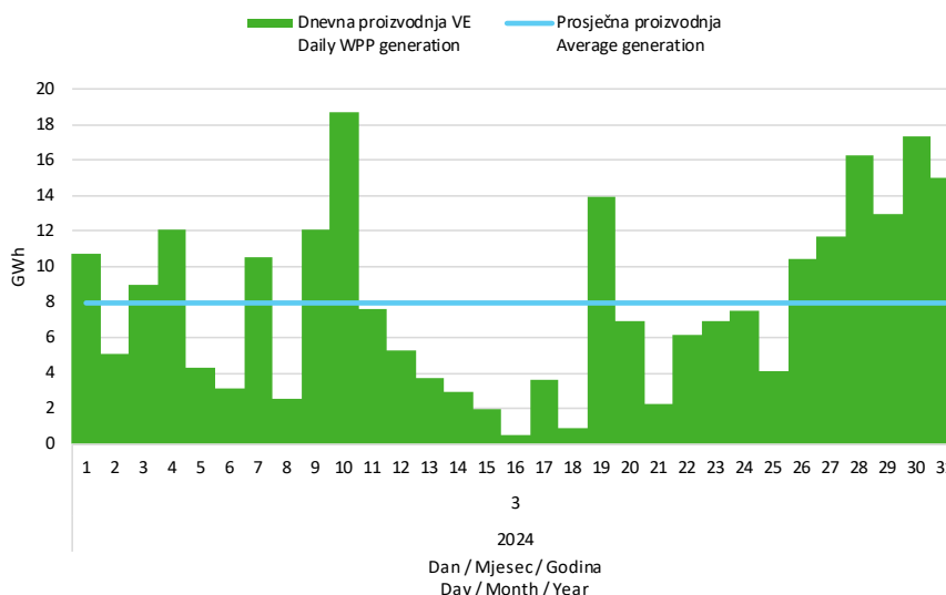
Slika 5 Dnevna proizvodnja svih vjetroelektrana u ožujku 2024. godine Figure 5 Daily generation of all wind power plants in March 2024
