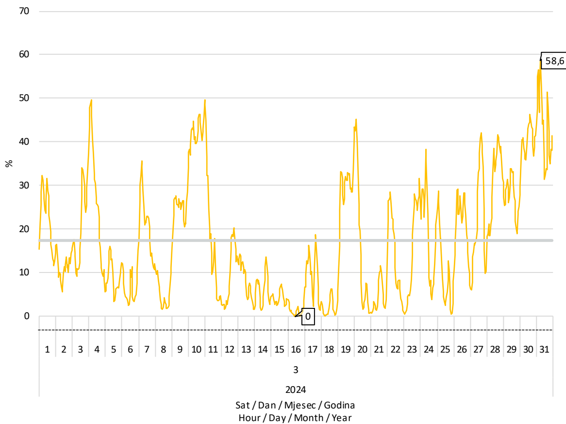
Slika 8 Udio proizvodnje vjetroelektrana u pokrivanju satnog opterećenja elektroenergetskog sustava u ožujku 2024. godine
