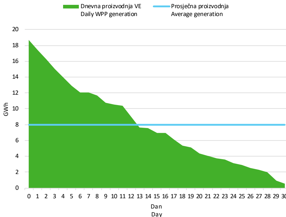
Slika 6 Krivulja trajanja dnevne proizvodnje vjetroelektrana u ožujku 2024. godine
